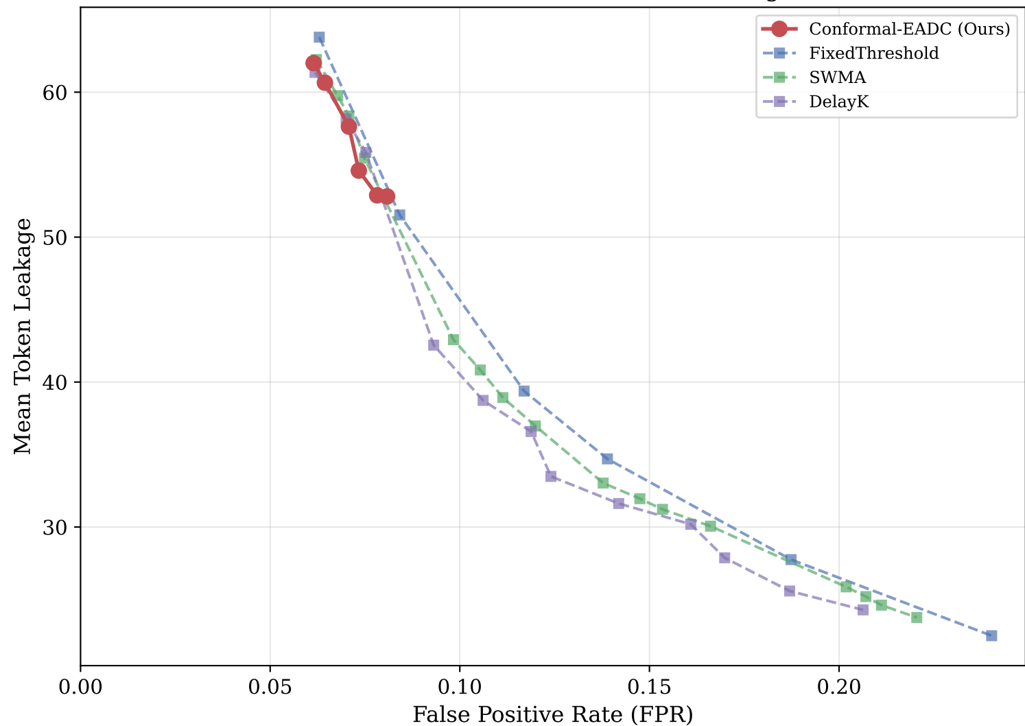
Pareto Frontier: FPR vs. Token Leakage
