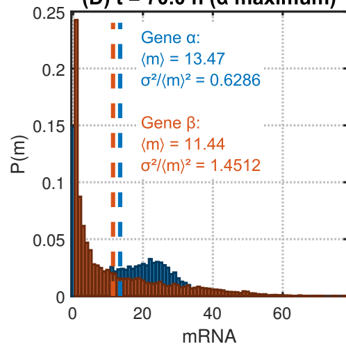
(D) t = 70.0 h ( \alpha maximum)
