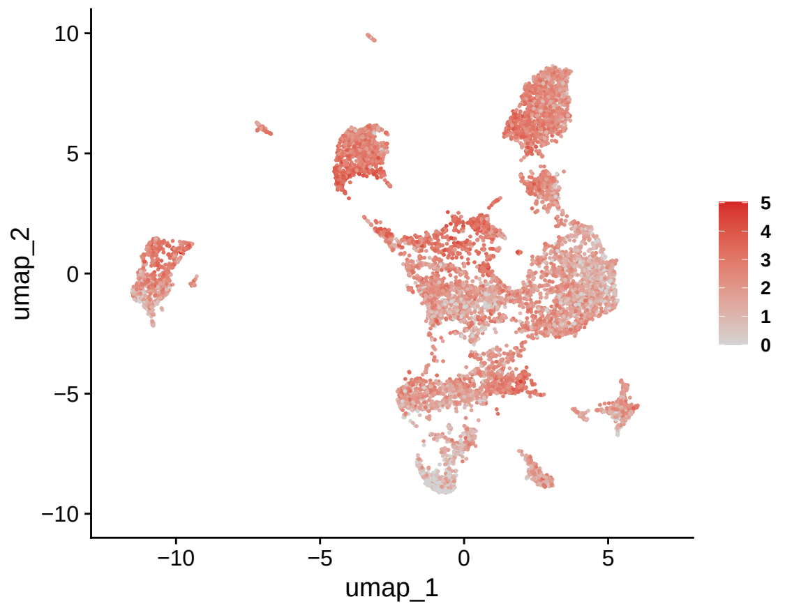
VIM
