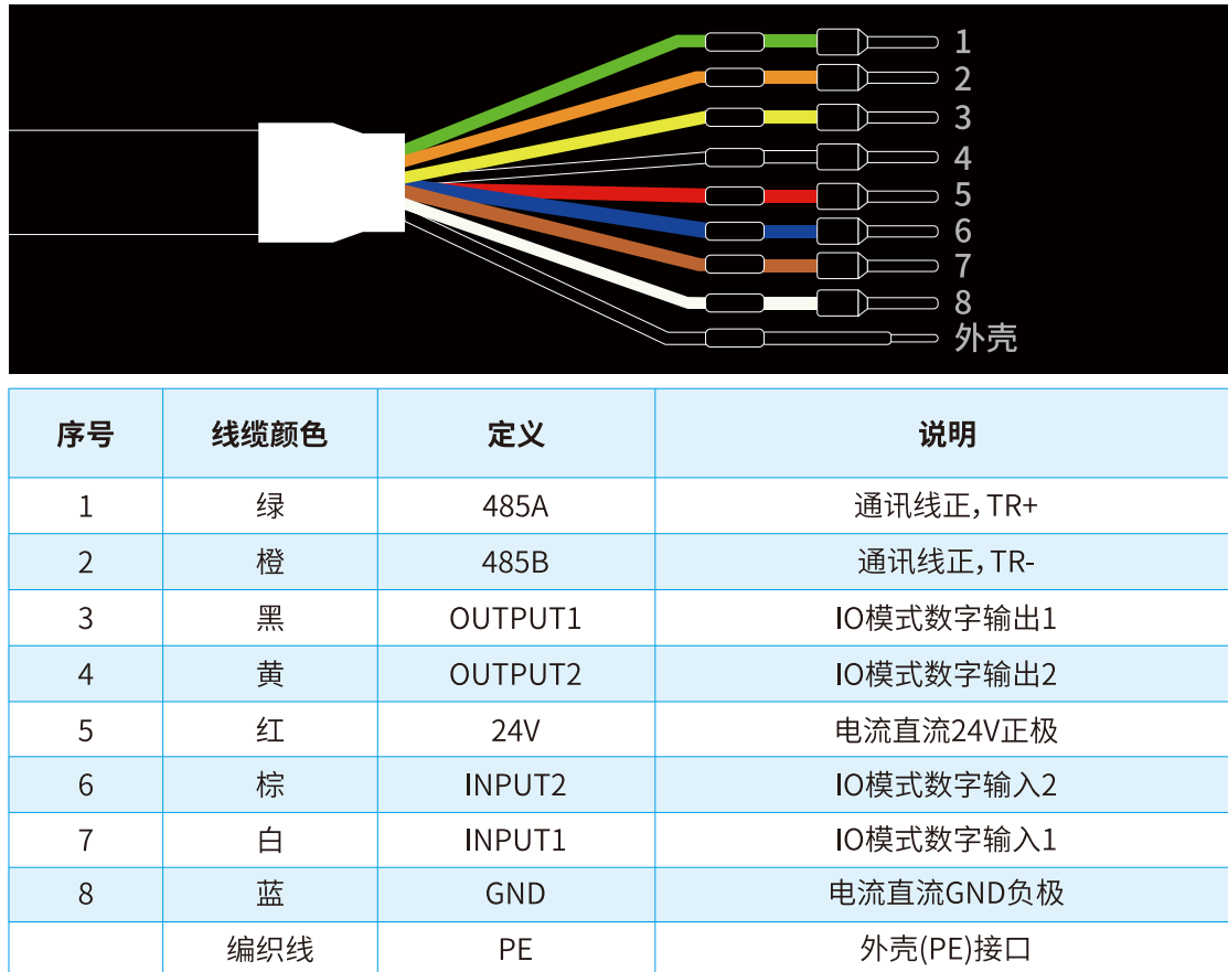
图1.1 线缆线标图
