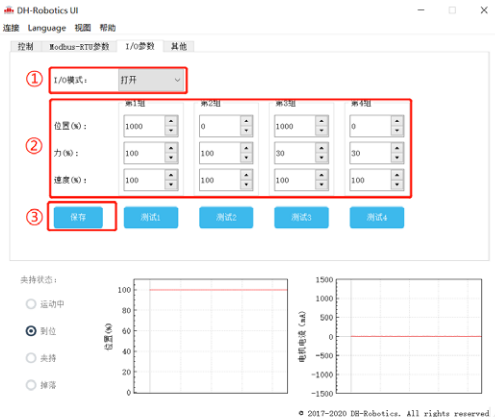
图3.1 IO设置
