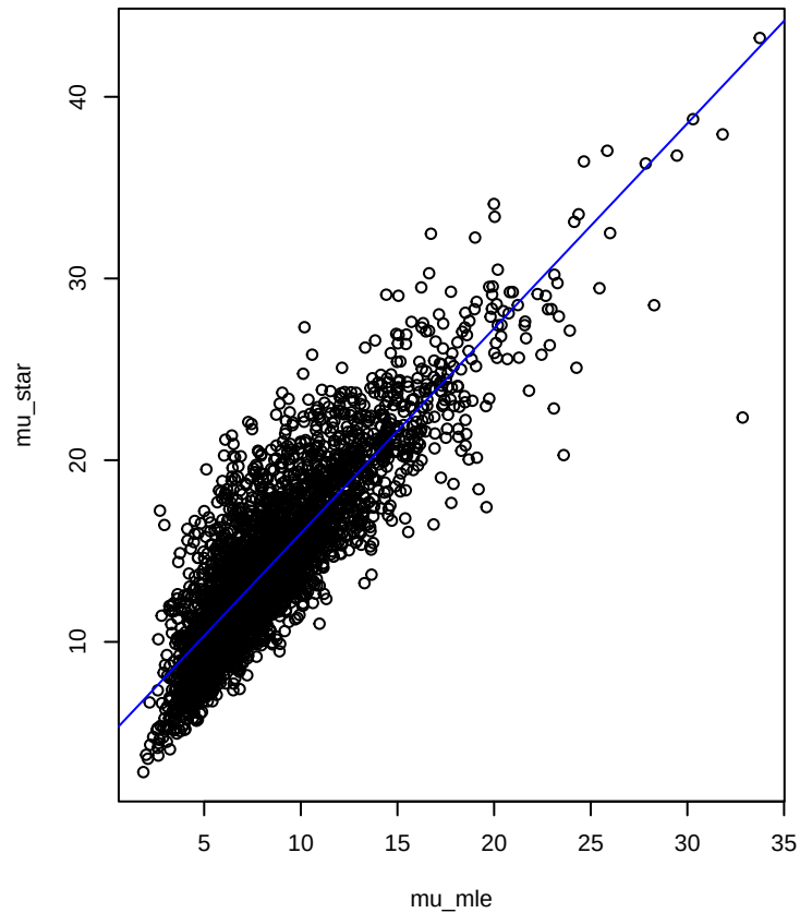
mu ( r=0.863 )
