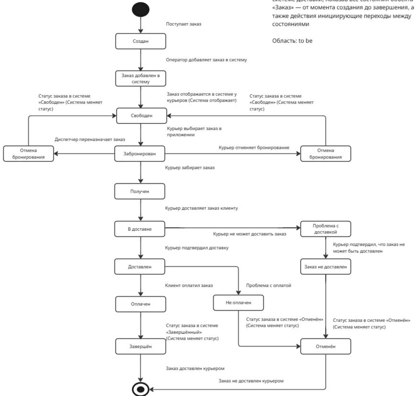
State diagram «Заказ в системе доставки»
