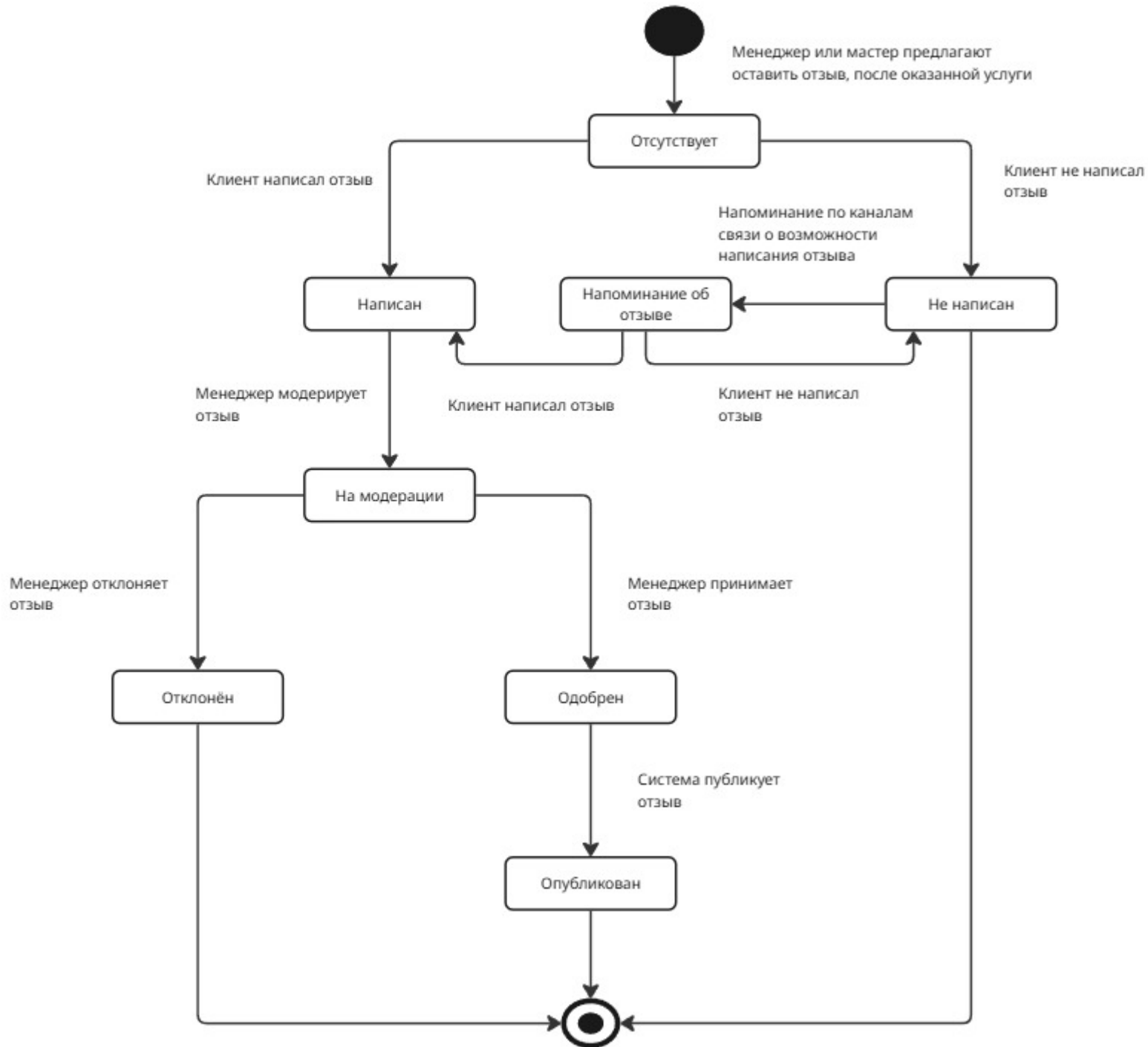
State diagram «Отзыв клиента»
