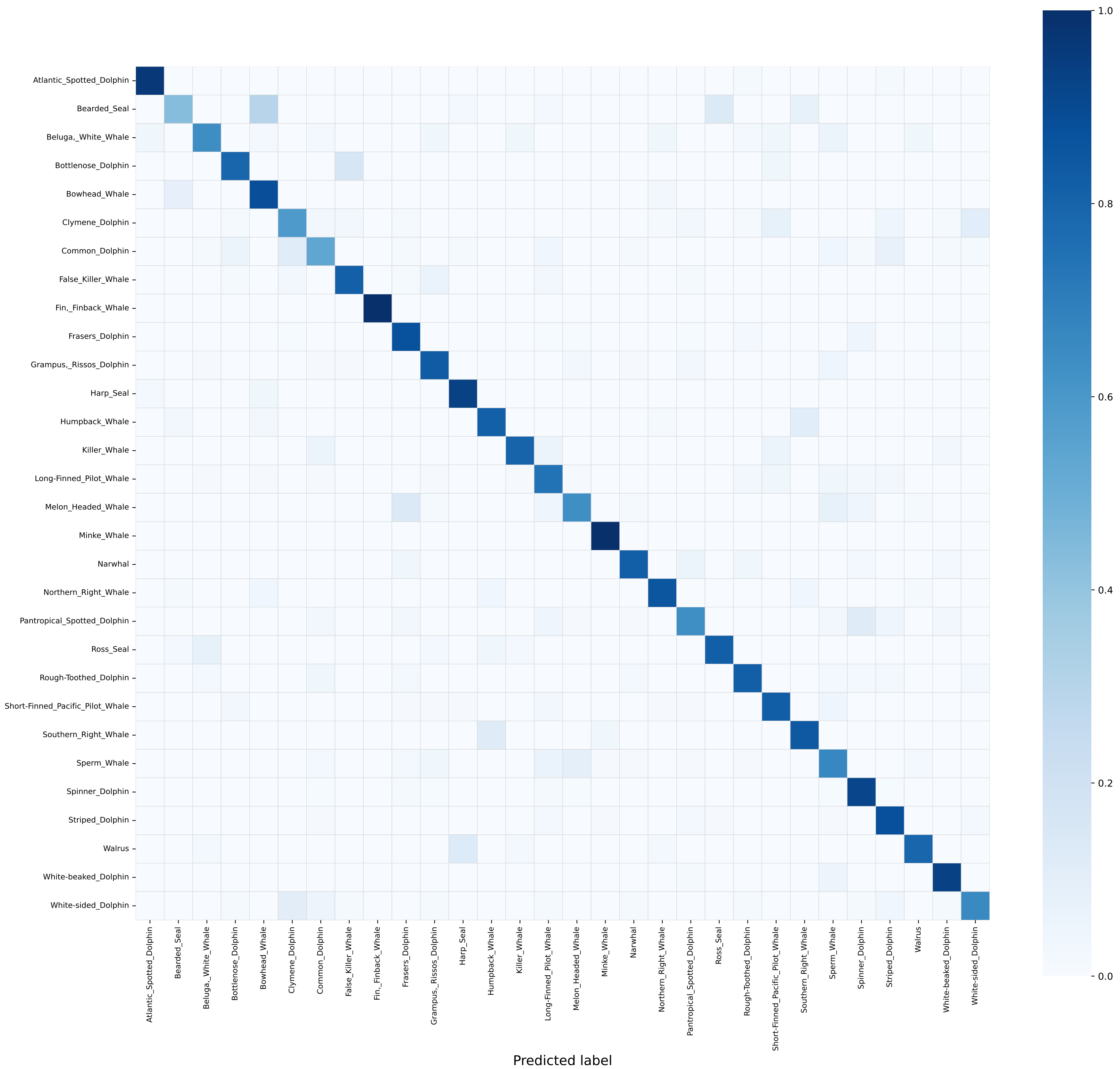
True label
