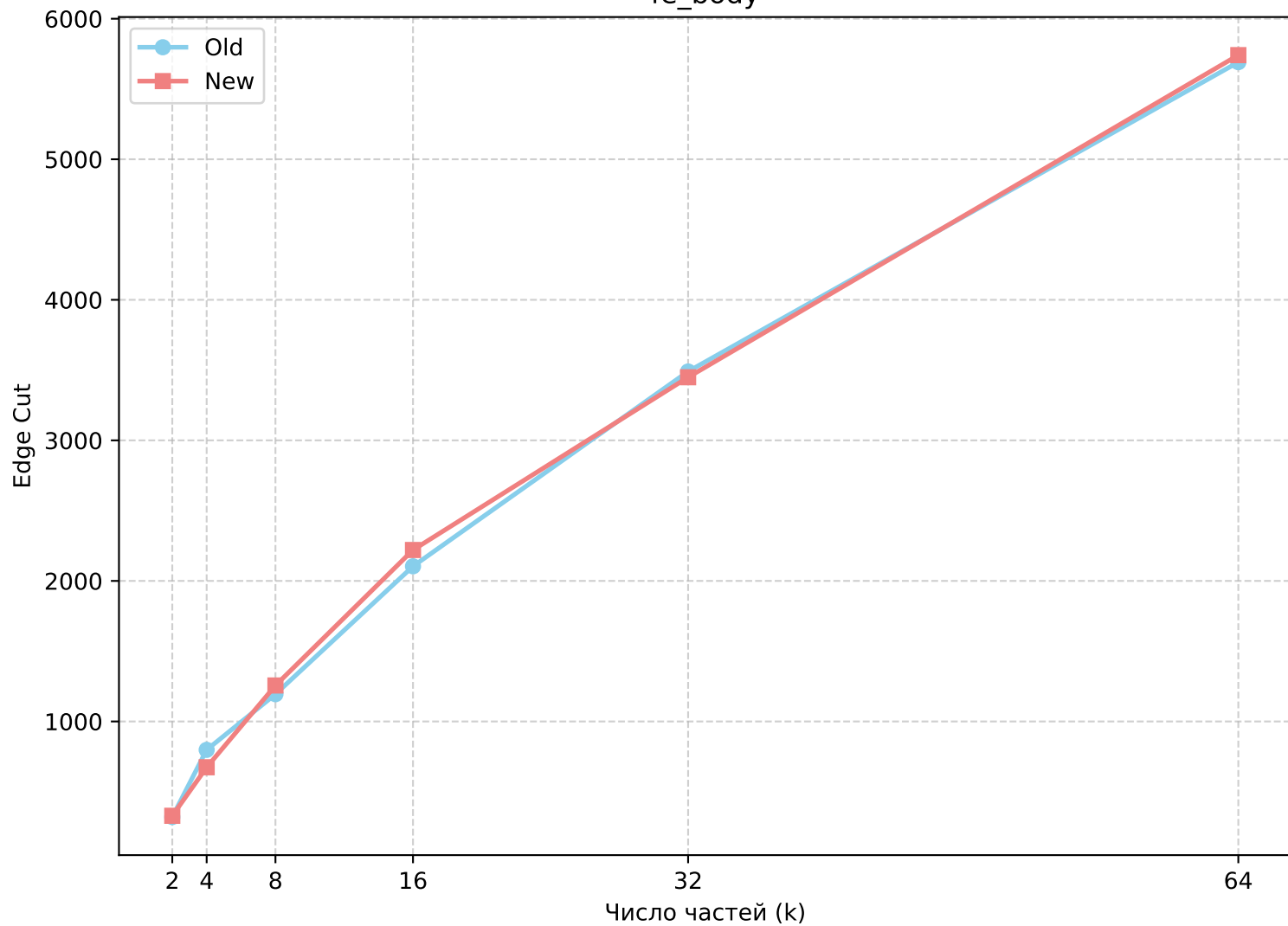
fe_body
