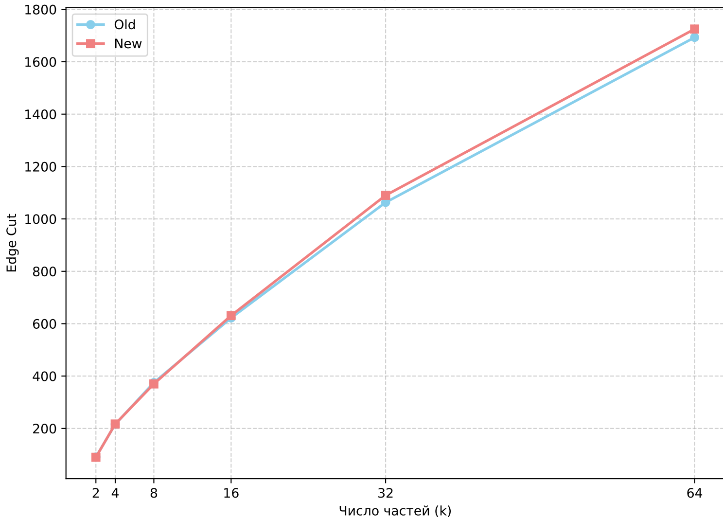
3elt
