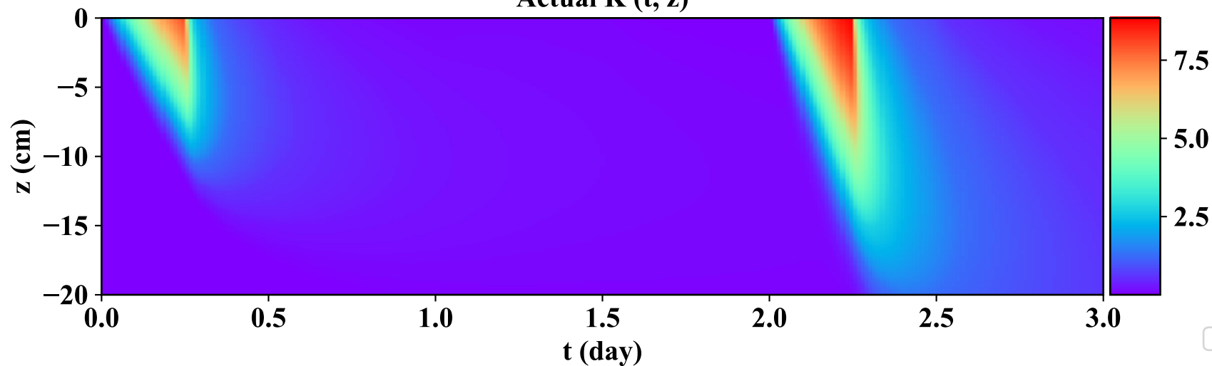
Actual K(t, z)
