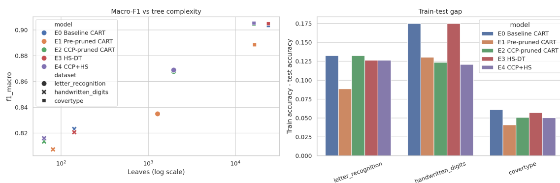
Hình 5.2: Quan hệ giữa macro-F1 và độ phức tạp của cây.
