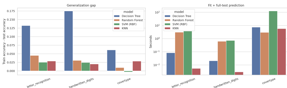
Hình 4.2: Train-test gap và thời gian chạy. Trục thời gian dùng thang logarithm.
