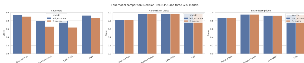
Hình 4.1: Accuracy và macro-F1 của bốn mô hình trên ba bộ dữ liệu.
