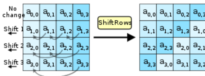
Hình 3.22. Hàm ShiftRows
