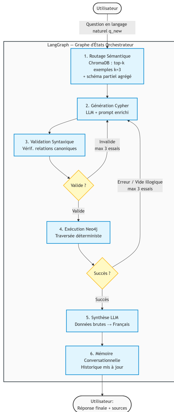
FIGURE 8 – Pipeline d'orchestration Text-to-Cypher-to-Answer avec routage sémantique dynamique et boucle de rétroaction corrective (LangGraph). Les nœuds (1) à (6) correspondent aux états du graphe LangGraph. L'étape (3) valide que les relations générées appartiennent exclusivement au vocabulaire canonique de l'ontologie aplatie. Les arêtes de rétroaction vers le nœud (2) matérialisent les cycles de correction, bornés à N_{\max} = 3 itérations.
