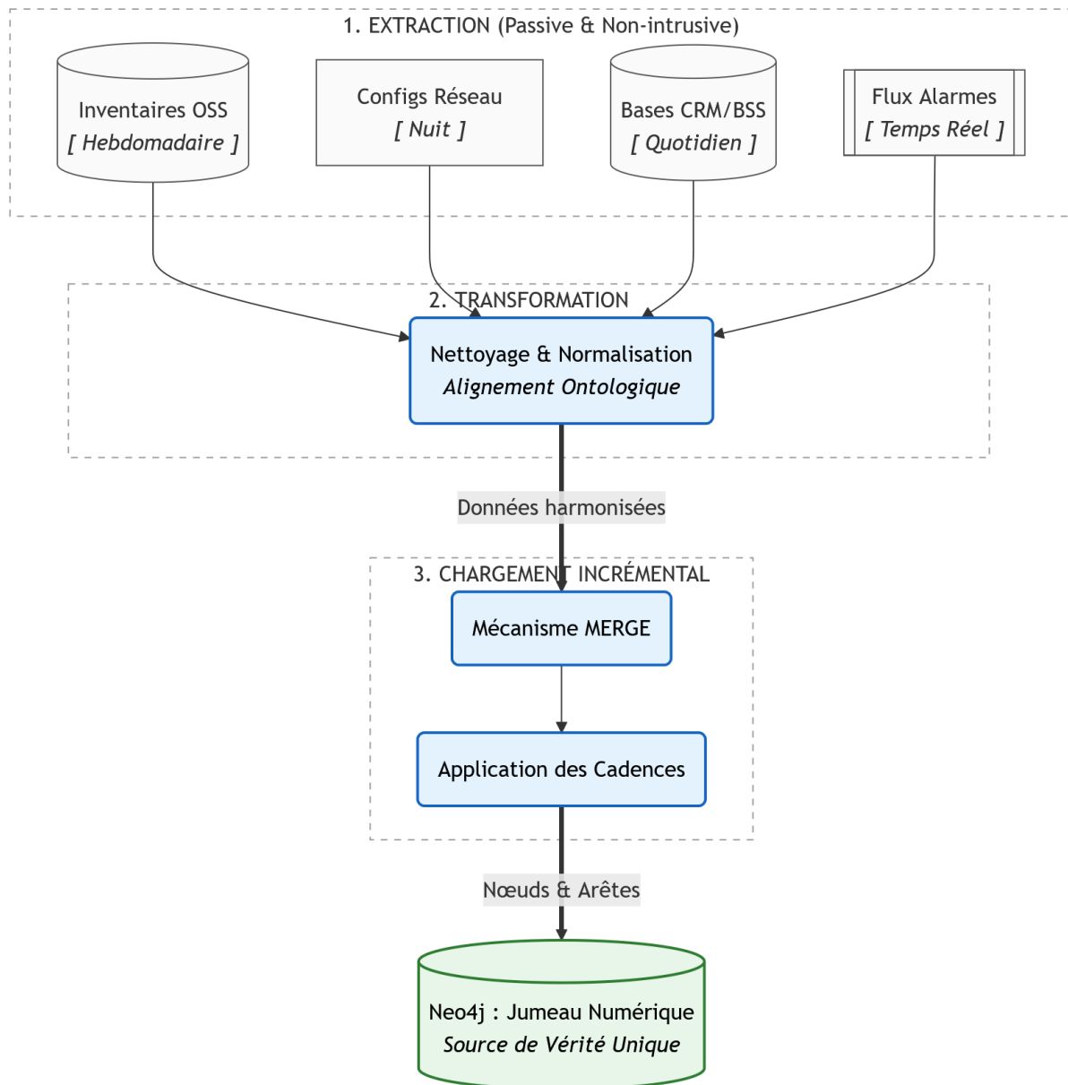
FIGURE 7 – Architecture fonctionnelle et flux de données du pipeline ETL vers le jumeau numérique
