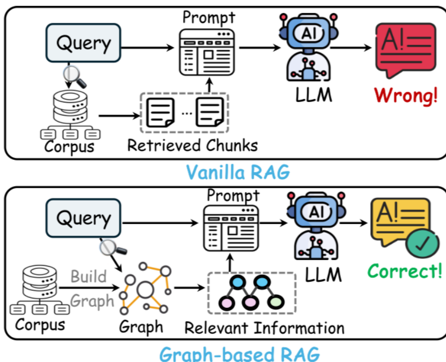
FIGURE 3 – Comparaison paradigmatique entre le RAG vectoriel ( Vanilla RAG ) et le GraphRAG. Là où l'approche classique récupère des fragments textuels isolés menant à des erreurs d'inférence, le GraphRAG construit et traverse une topologie explicite pour fournir au LLM un contexte relationnel structuré, garantissant l'exactitude du raisonnement multi-sauts.
