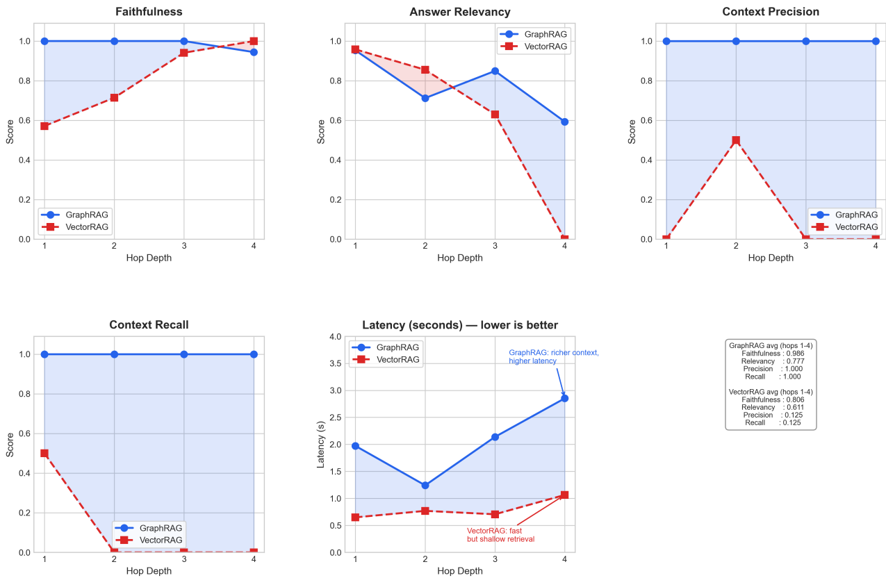
FIGURE 9 – Visualisation empirique du compromis ( trade-off ) : le GraphRAG maintient une exactitude topologique parfaite ( CR = 1,00 ) au prix d'une augmentation maîtrisée de la latence (inférieure à 3 secondes), tandis que le RAG vectoriel s'effondre structurellement dès k = 2 .
