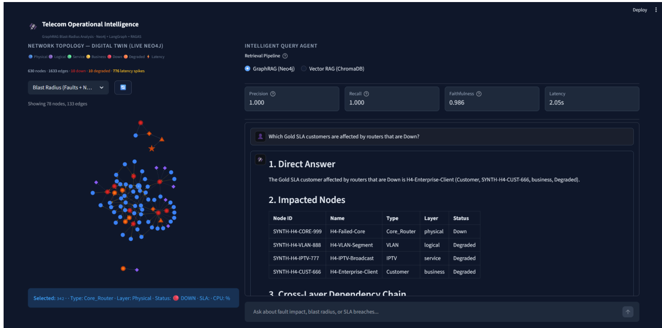
FIGURE 10 – Interface de diagnostic GraphRAG : génération du rapport d'impact complet ( blast radius à 4 sauts) pour une défaillance de routeur de cœur. Chaque ligne du rapport est tracée jusqu'au nœud Neo4j source.
