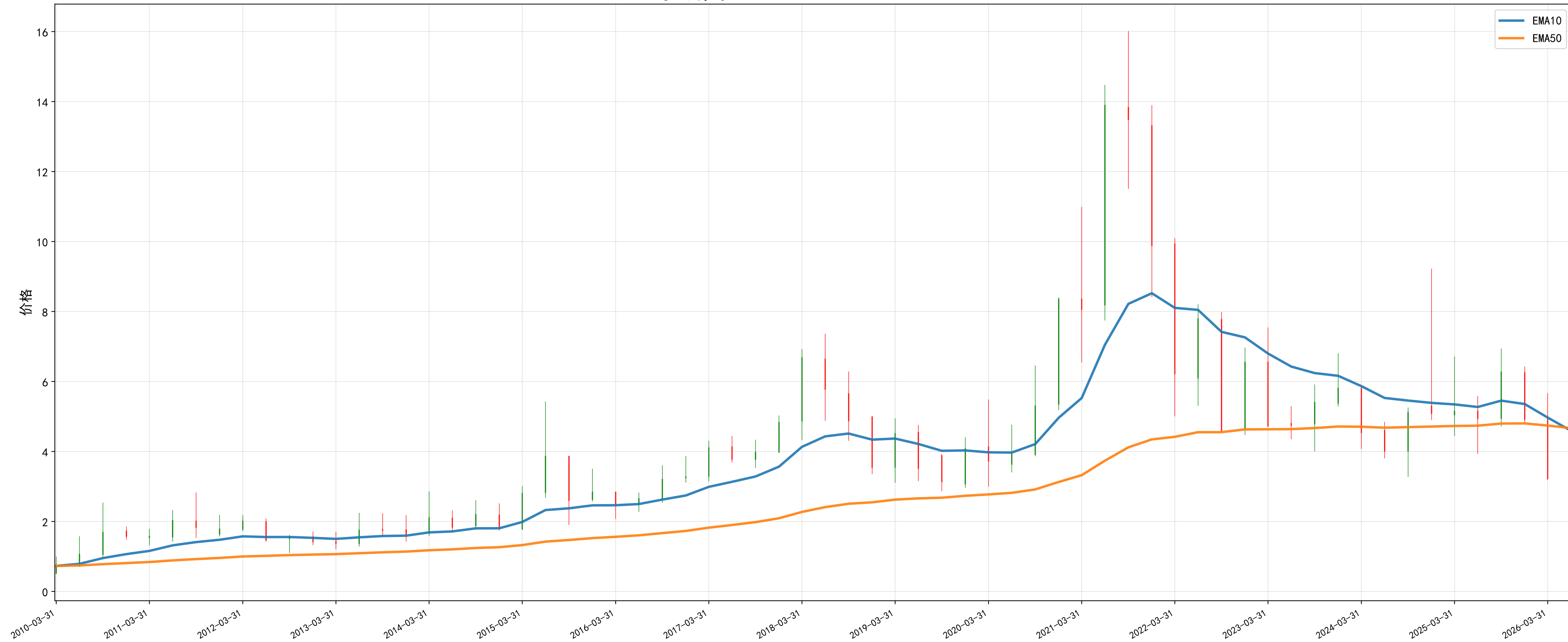
00354 季线图 - 2010-03-31 至 2026-06-30
