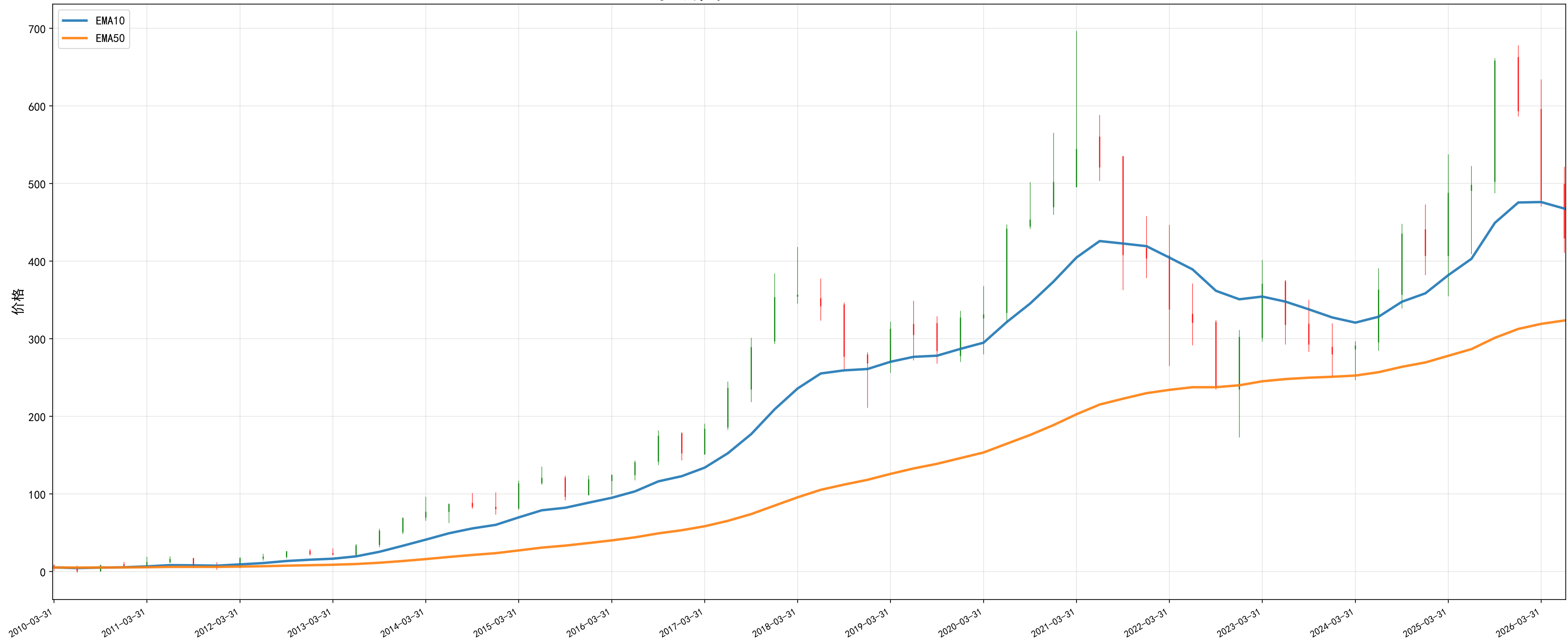
00700 季线图 - 2010-03-31 至 2026-06-30
