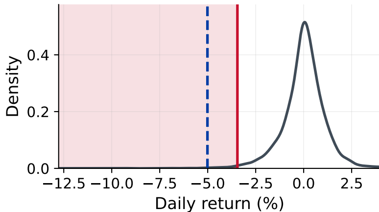
S&amp;P 500, 6791 days
