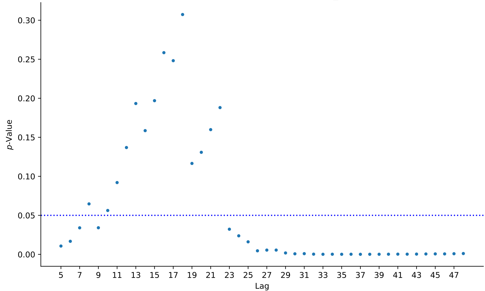
Ljung-Box P-values: (3,0,0)(0,1,1)_12
