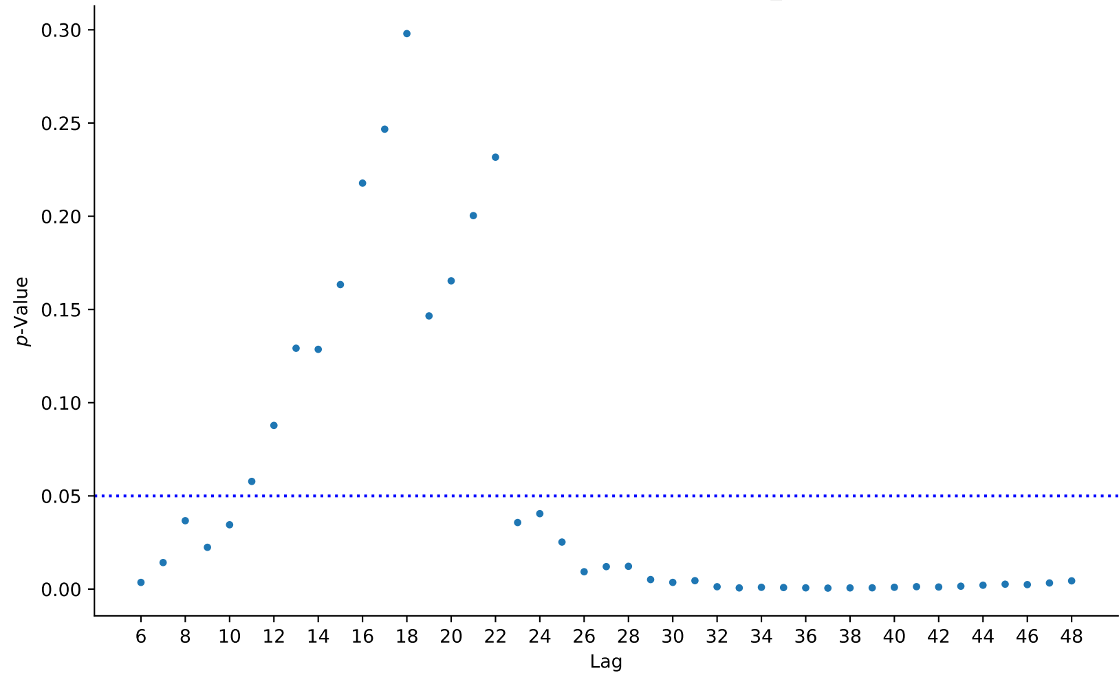
Ljung-Box P-values: (3,0,0)(2,1,0)_12
