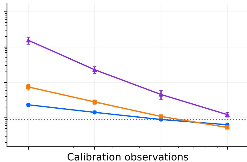
(d) Student-t(5): state-dependent distortion
