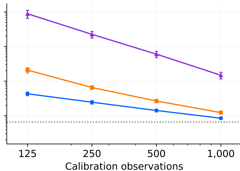
(d) Student-t(5): state-dependent distortion
