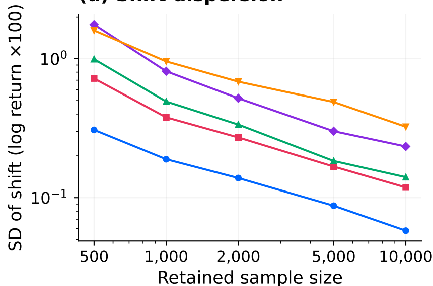
(d) Shift dispersion
