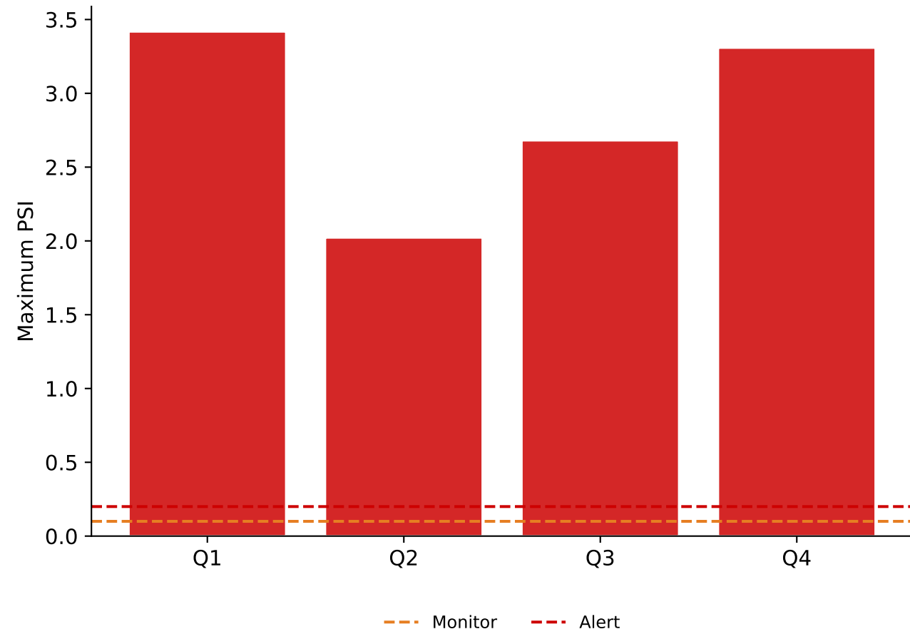
Data Drift (PSI)
