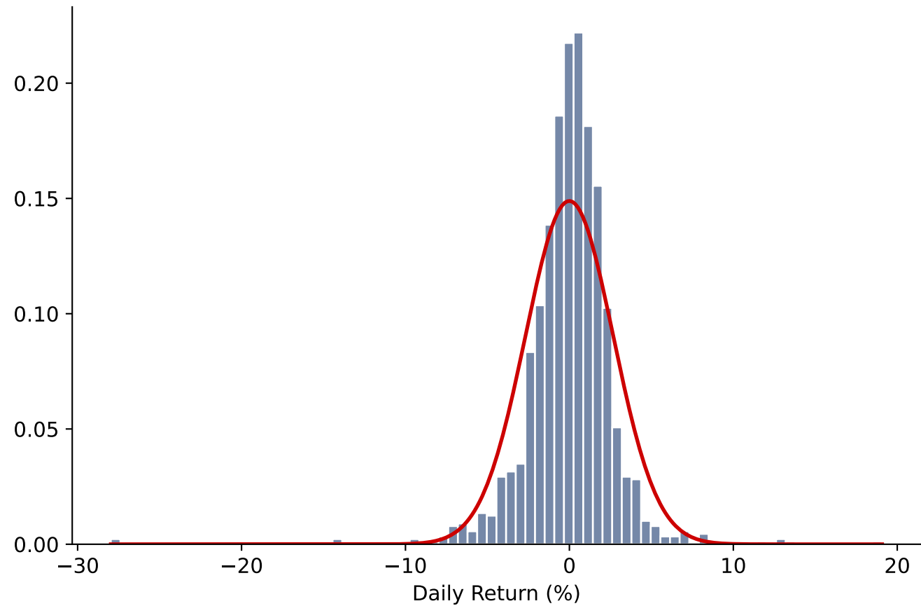
Brent Oil Returns (Kurtosis: 22.5)
