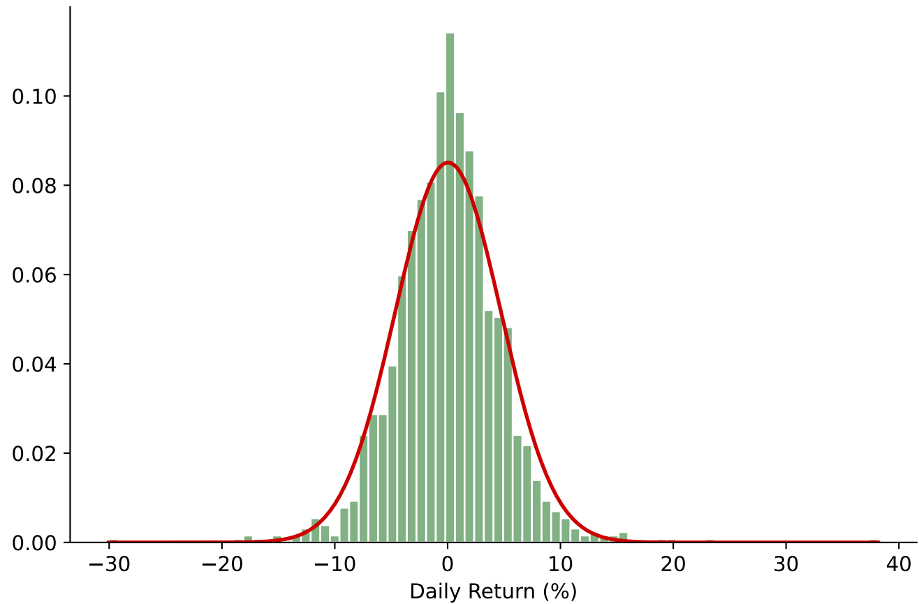
Natural Gas Returns (Kurtosis: 8.1)
