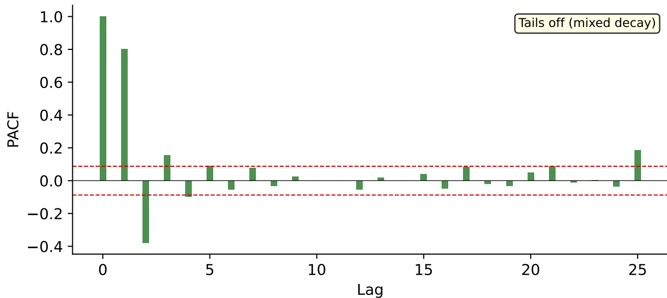
ARMA(1,1) — PACF
