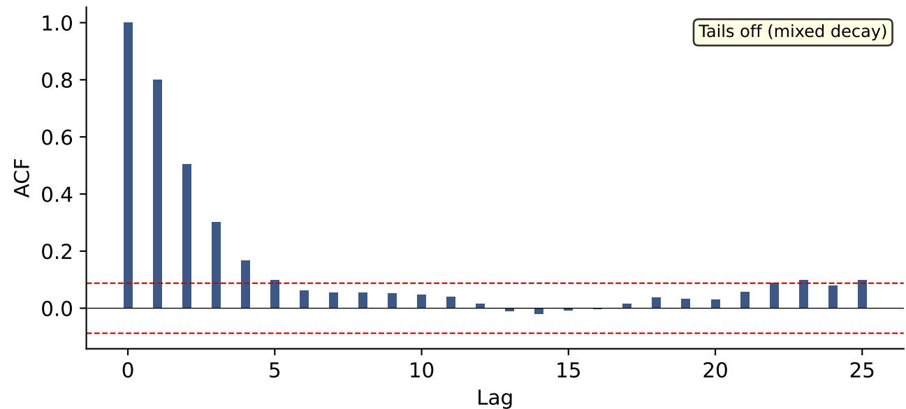
ARMA(1,1) — ACF
