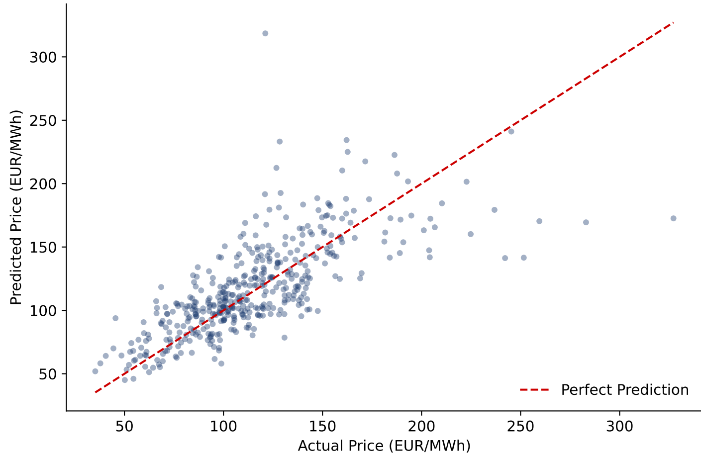
Scatter: Actual vs Predicted
