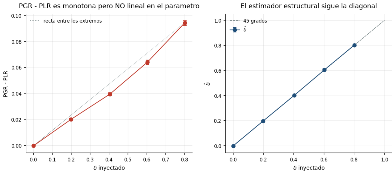
Figura 6: No linealidad
