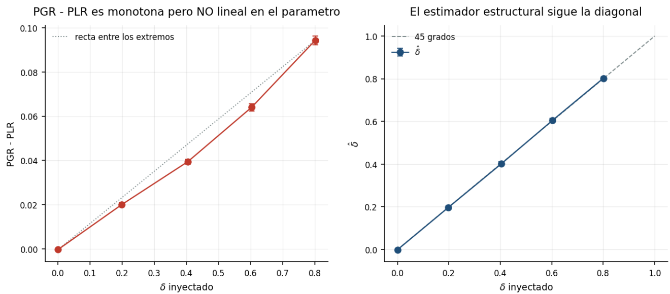
Figura 6: No linealidad
