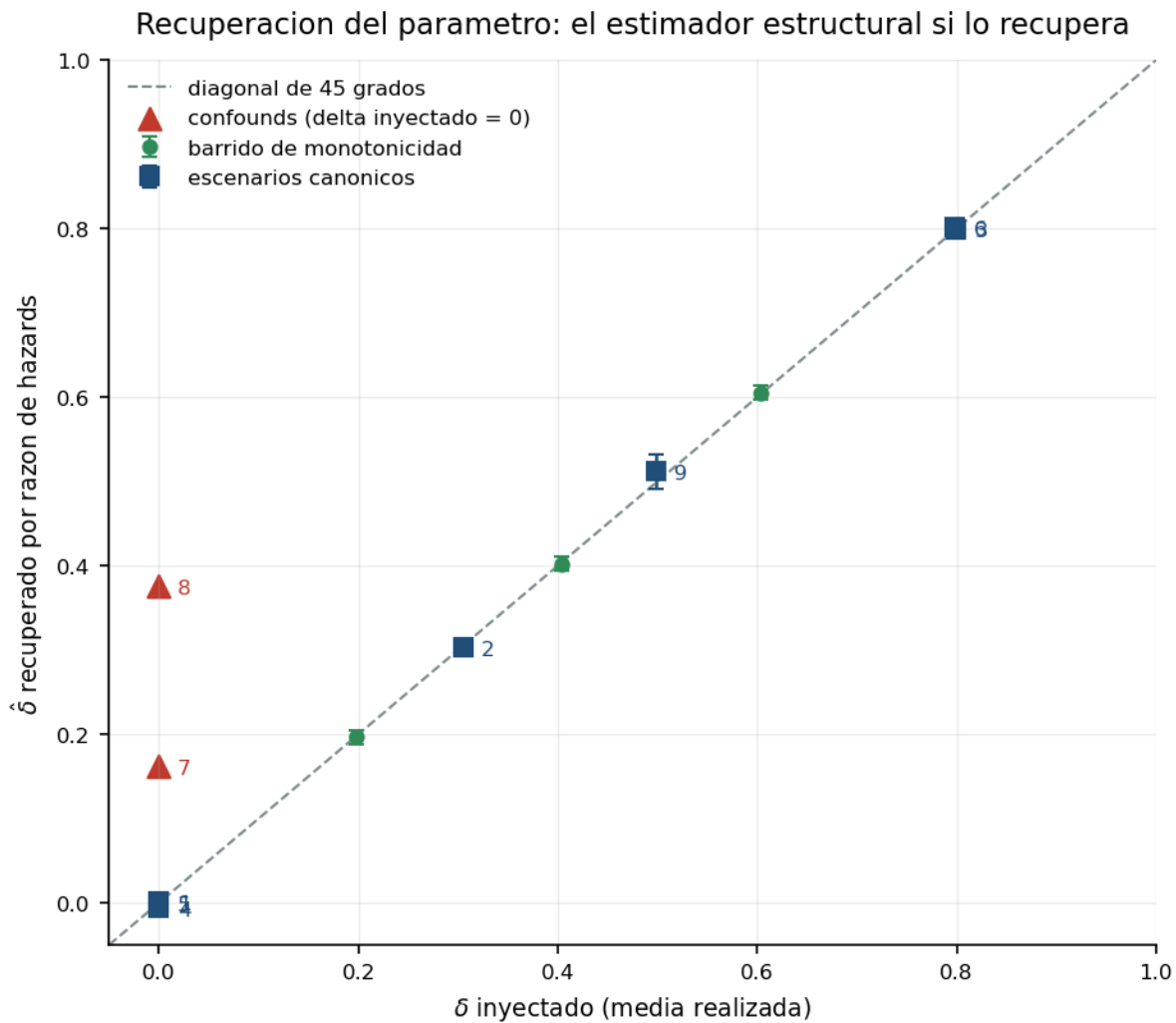
Figura 4: Recuperación de delta
