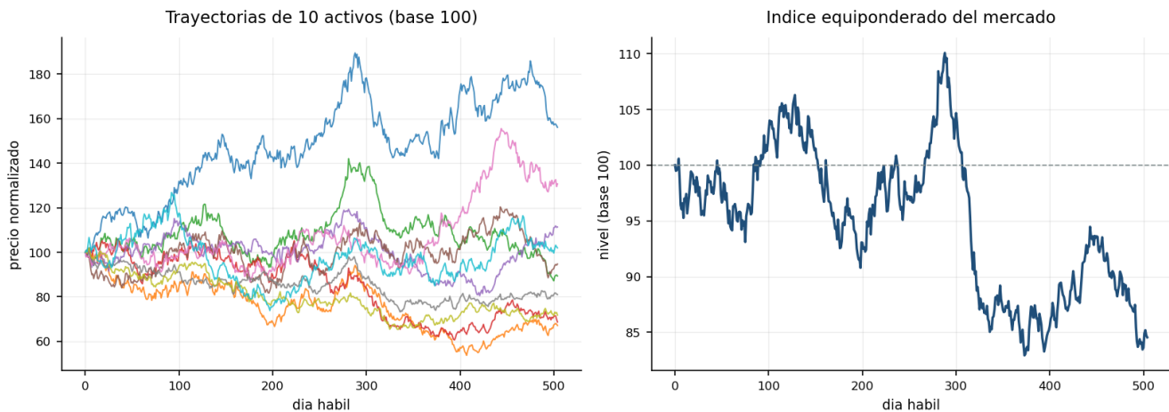
Figura 1: Trayectorias de precios
