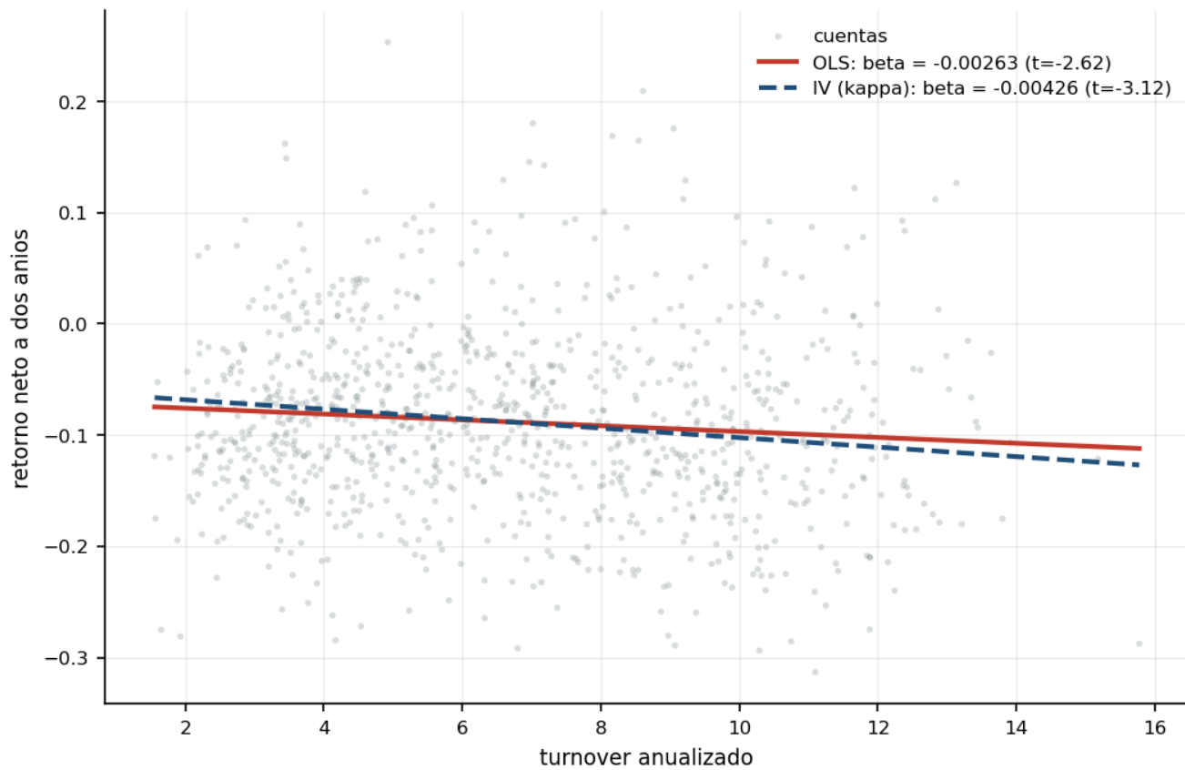
Figura 8: Turnover contra retorno
