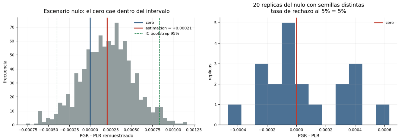
Figura 5: Bootstrap del nulo
