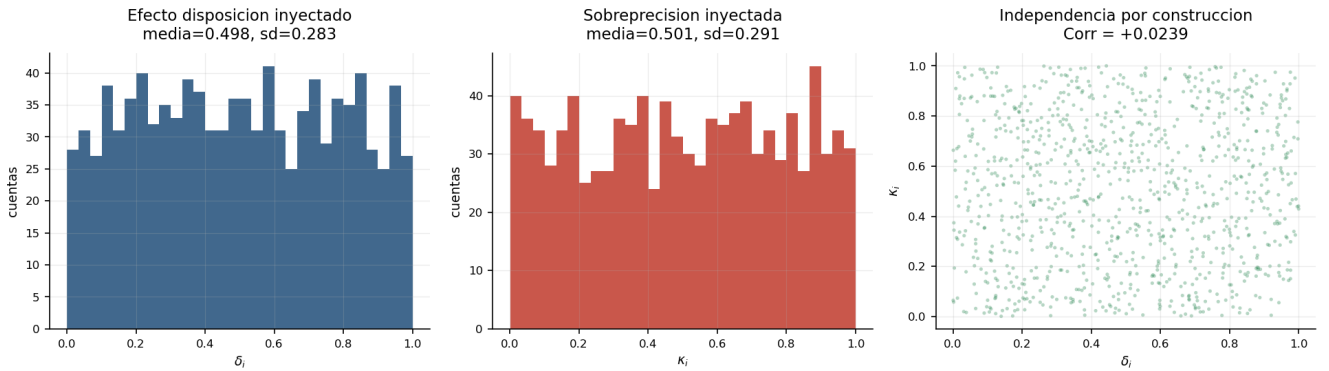
Figura 2: Distribución de delta y kappa
