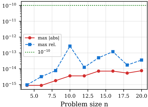
Equivalence (200 random x per n)
