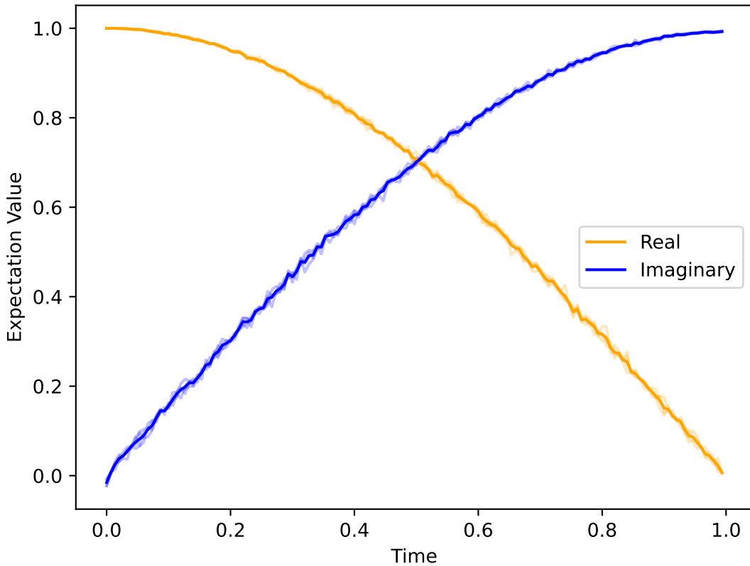
Expectation Value with \Delta t=0.006666666666666667
