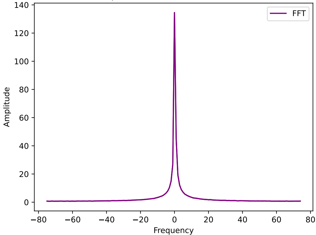
Fourier Transform of Expectation Value with \Delta t=0.006666666666666667
