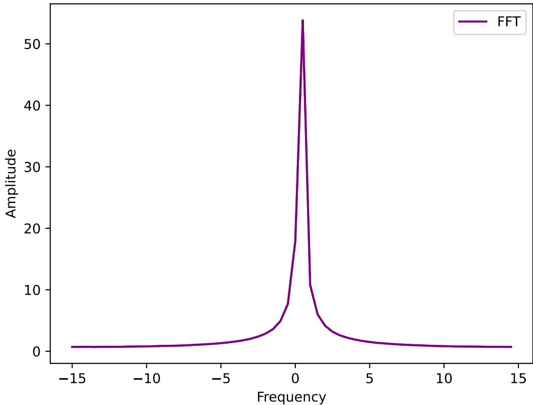
Fourier Transform of Expectation Value with \Delta t=0.03333333333333333
