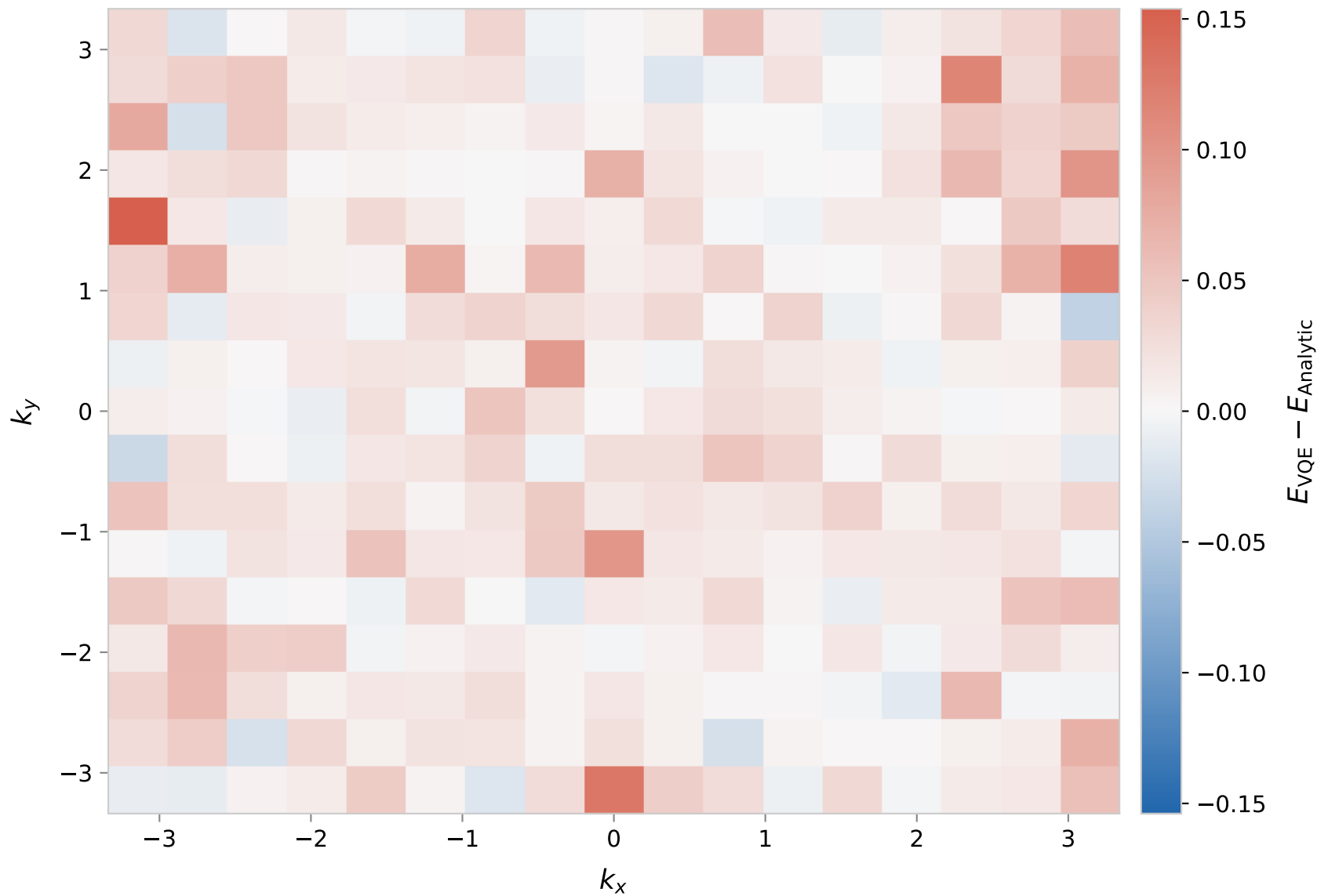
Haldane, VQE – Analytic
