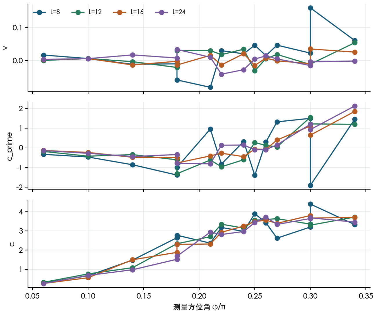
图 8. 区分面积律、对数与平方对数行为的弧模型系数。 解读边界: 解读受有限宽度和预先声明拟合窗口约束。
