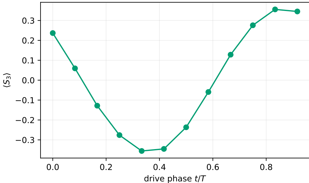
N=3 reflection-even periodic state — PT-TEMPO
