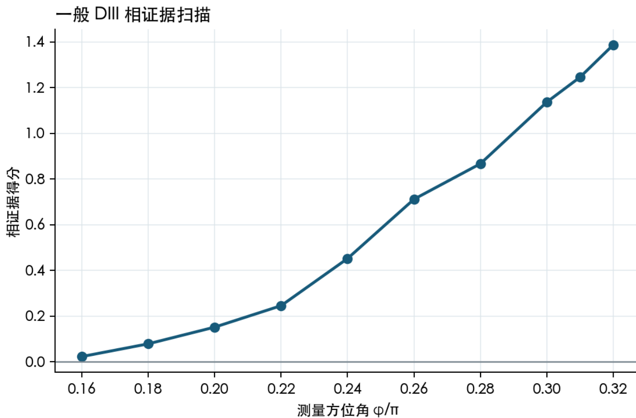
图 7. 一般 DIII 粗扫描证据与选定细化括区。 解读边界：解读受有限宽度和预先声明拟合窗口约束。
