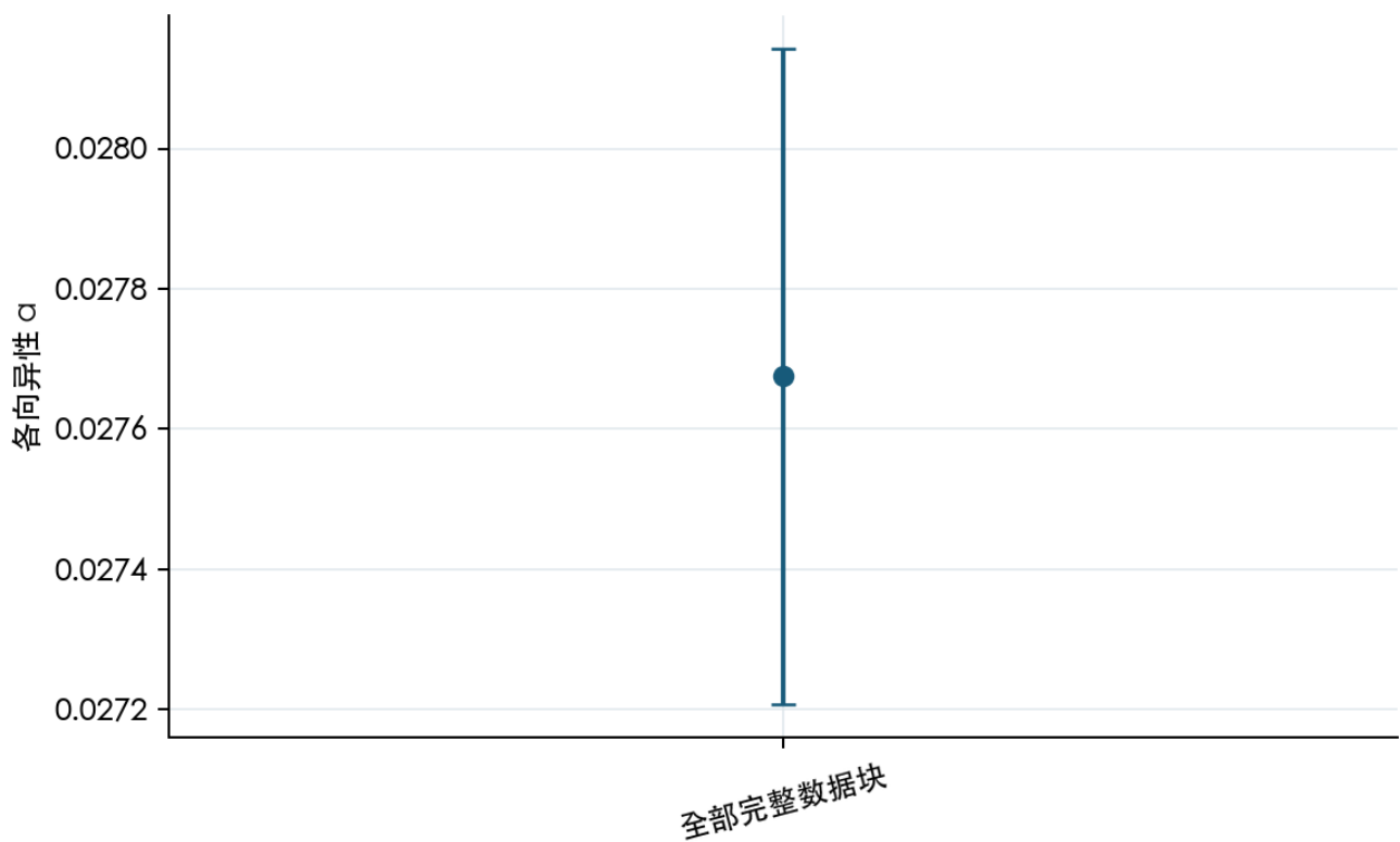
图 17. 各向异性在预先声明分析窗口间的稳定性。 解读边界: 解读受有限宽度和预先声明拟合窗口约束。
