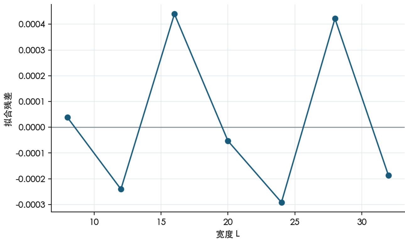
图 16. Casimir 有限尺寸拟合残差。 解读边界: 解读受有限宽度和预先声明拟合窗口约束。
