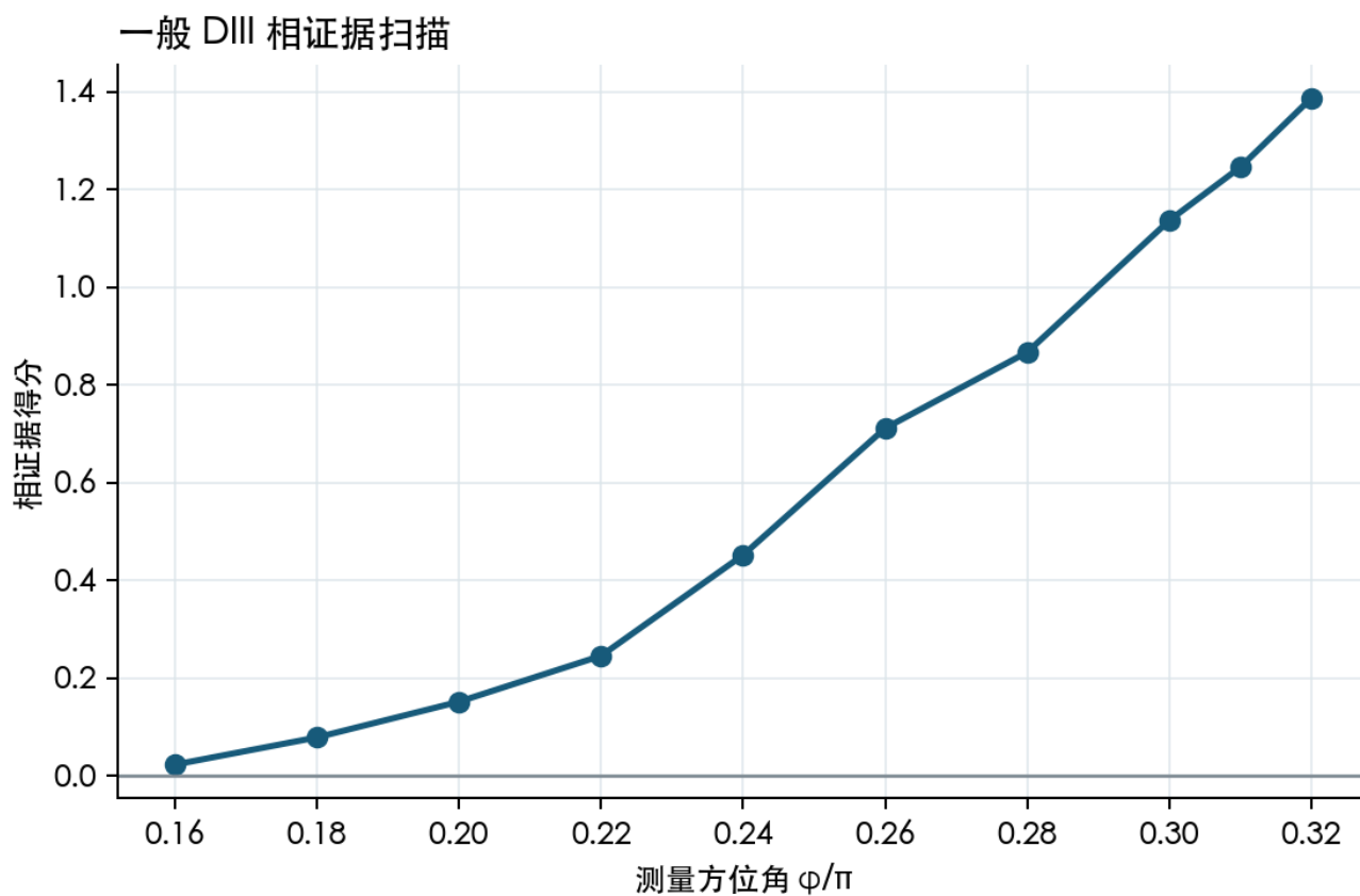
图 3. 一般 DIII 粗扫描证据与选定细化括区。 解读边界: 解读受有限宽度和预先声明拟合窗口约束。
