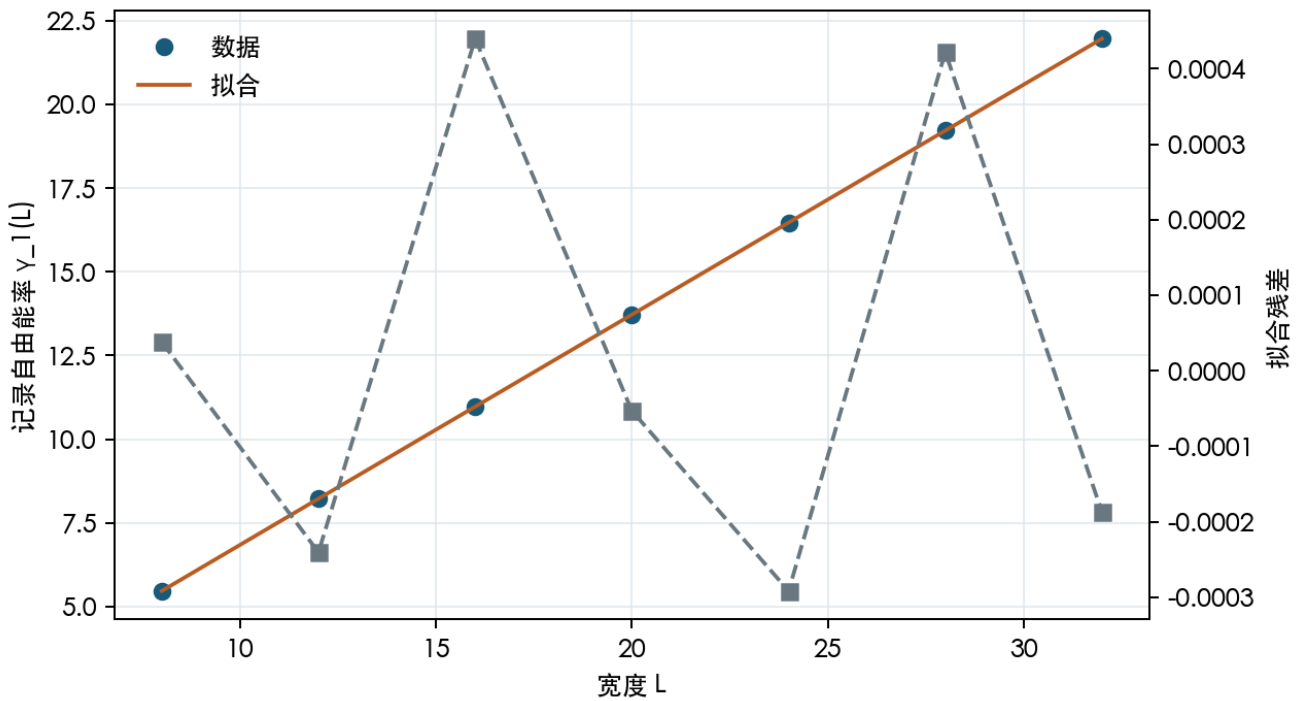
图 15. 含残差的 Casimir 有限尺寸拟合。 解读边界: 解读受有限宽度和预先声明拟合窗口约束。
