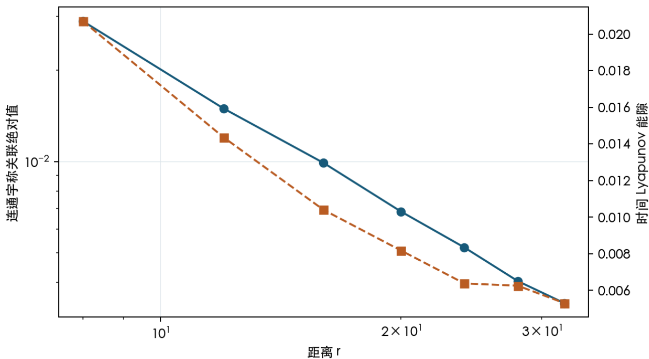
图 11. 空间宇称衰减与时间 Lyapunov 能隙。 解读边界: 解读受有限宽度和预先声明拟合窗口约束。
