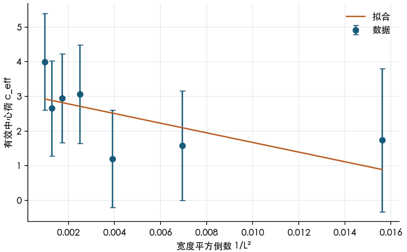
图 14. 纠缠有效中心荷的有限尺寸外推。 解读边界: 解读受有限宽度和预先声明拟合窗口约束。
