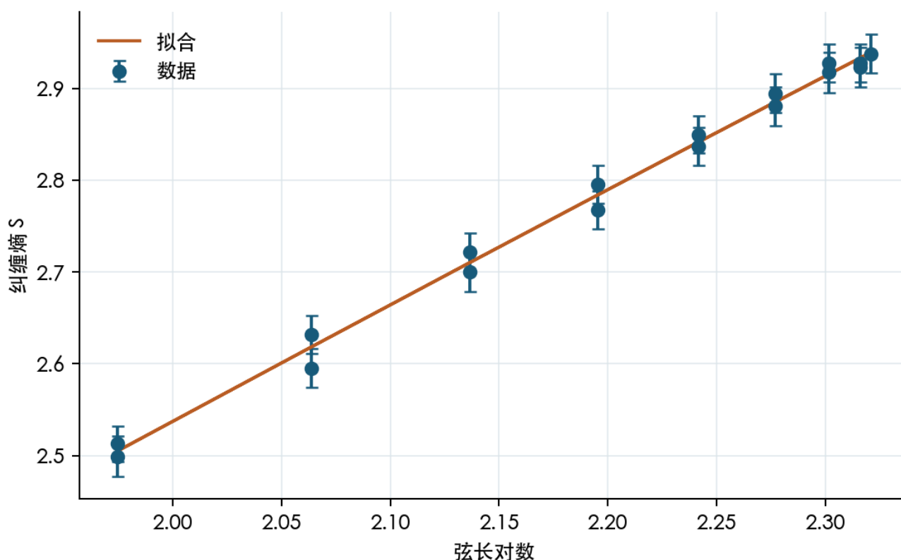
图 13. 选定 DIII 角度下纠缠熵对周期弦长的拟合。 解读边界：解读受有限宽度和预先声明拟合窗口约束。
