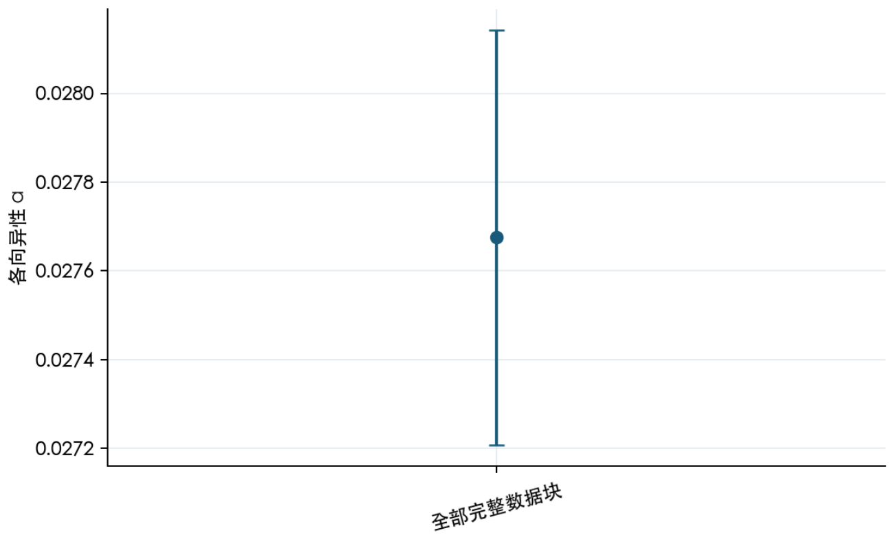
图 12. 各向异性对分析窗口的敏感性。 解读边界: 解读受有限宽度和预先声明拟合窗口约束。
