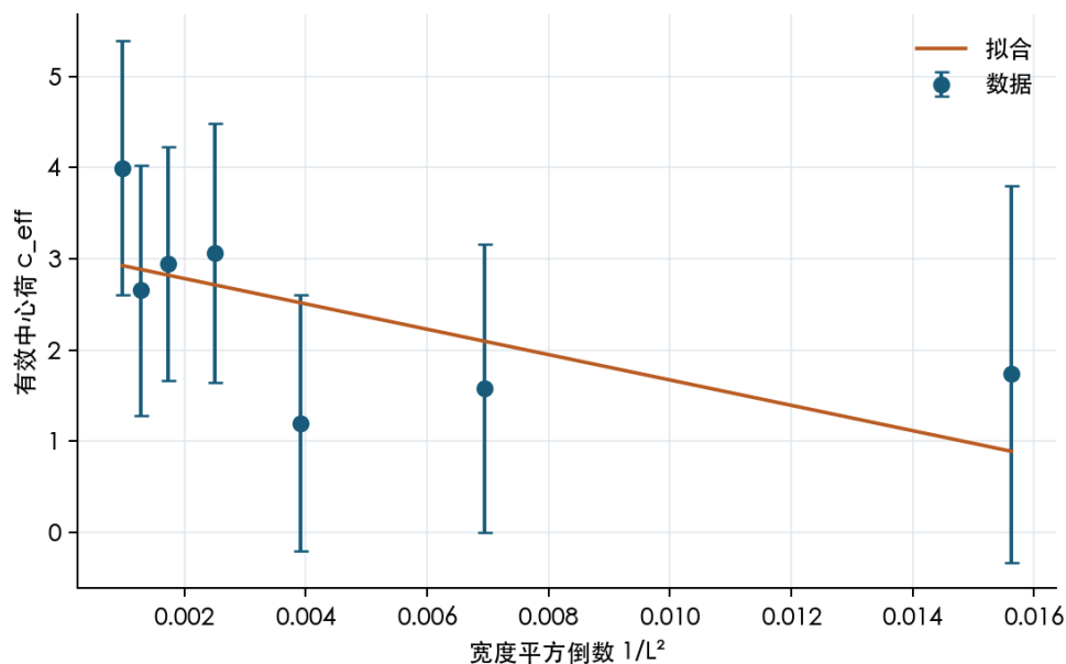
图 23. 截距为 3.060740, 95% 区间为 [1.571634, 4.549845]。解读边界: 区间很宽, 原因是逐宽度斜率噪声较大且有限尺寸依赖显著。
