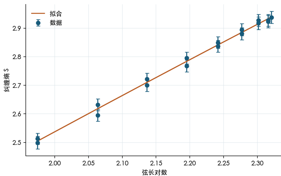
图 22. 中央区间纠缠数据与用于提取 c_{\text{eff}}(L) 的共形弦长形式比较。解读边界: 弦长曲线视觉上平滑, 不能消除跨宽度外推误差, 也不能单独证明 DIII 临界点。
