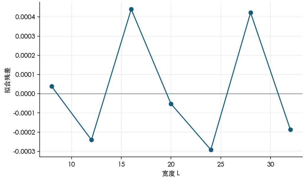
图 25. 残差结构用于检验所选修正族能否解释观测到的宽度依赖。解读边界: 小残差不能补救不稳定的各向异性标定。
