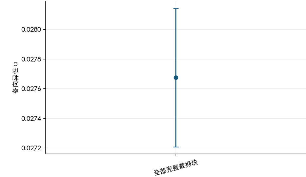
图 26. 冻结 \alpha 估计为 0.027675；稳定性门控通过：否。解读边界：窗口敏感性直接传播到 c_{\text{eff}}^{\wedge}C ，因此它是发布所必需的门控。
