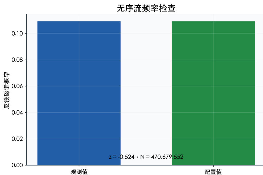
图 11. 观测负键概率与配置 p 的比较。解读边界: 边缘频率不能检验 RNG 的全部时空相关。
