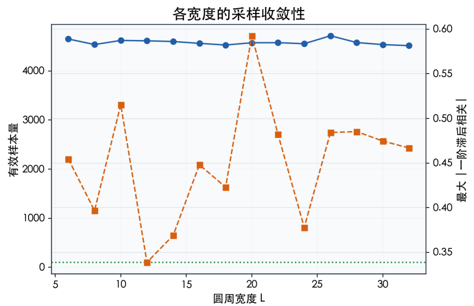
图 14. 各宽度 ESS 与一阶滞后相关。解读边界: ESS 不诊断有限尺寸模型偏差。
