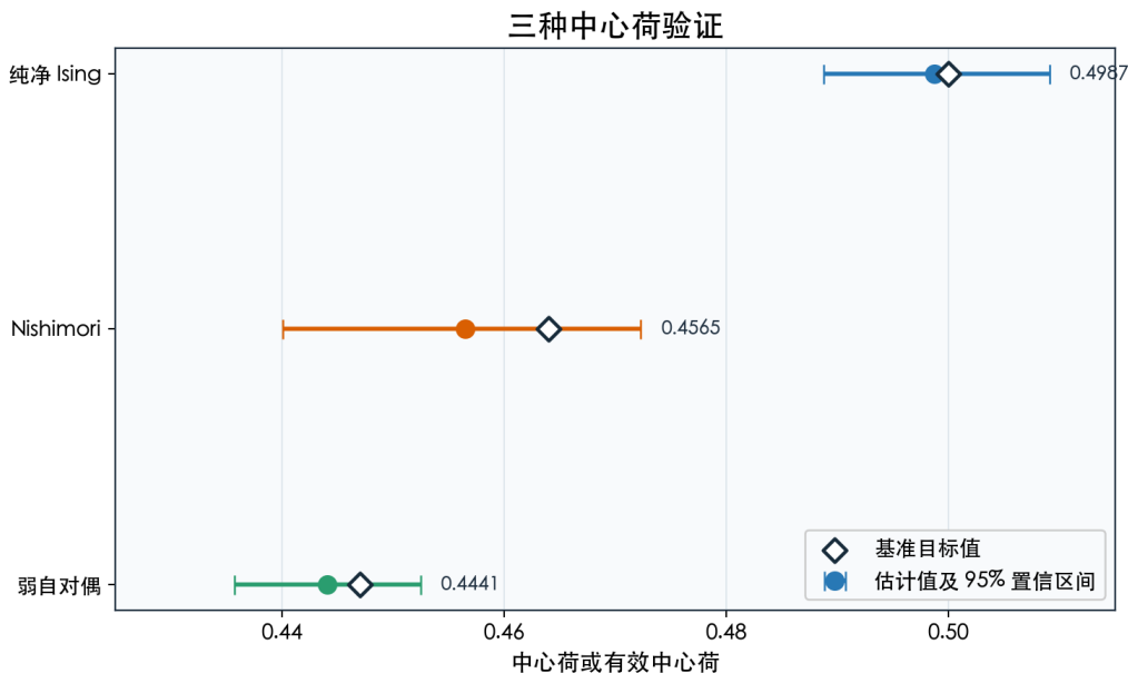
图 1. 三个中心荷估计及 95% 置信区间与各自基准值的并列比较。解读边界：
