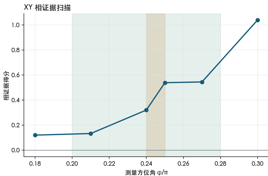
图 22. 验证扫描：冻结 XY 括区为 [0.24, 0.25] ，位于声明的参考窗口内。解读边界：该图只验证特殊 D 类线上的实现，不能据此证明一般 DIII 转变。
