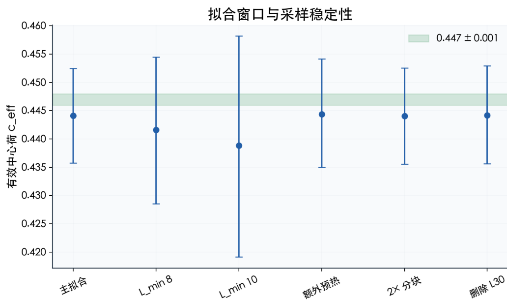
图 16. 比较最小宽度、预热、块长和删宽度变体。解读边界: 已测变体不包含所有可能修正。
