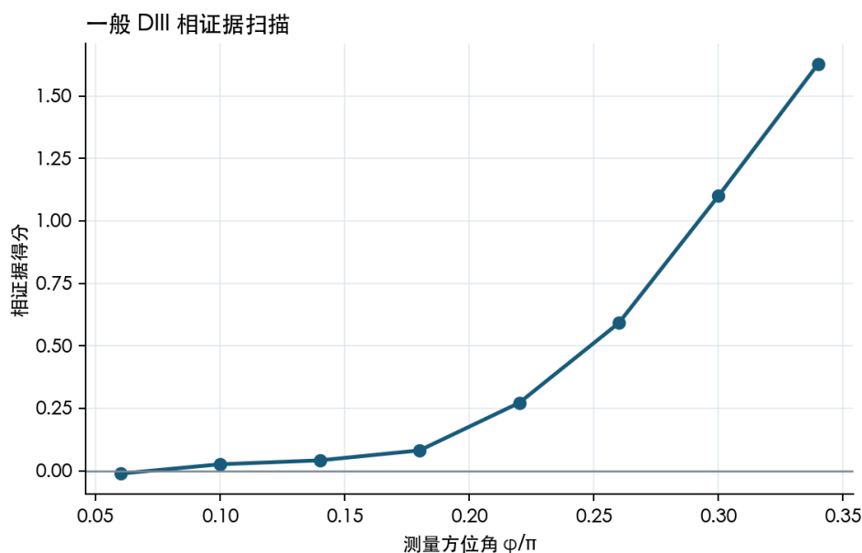
图 23. 探索性一般 DIII 扫描。分数随网格平滑变化，但没有相邻点满足完整的持续相反相证据规则。解读边界：该分数是复合有限尺寸诊断，不是中心荷，也不是零点具有普适意义的独立序参量。
