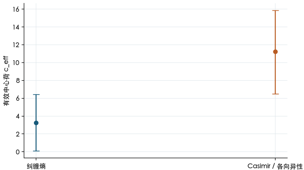
图 18. 独立的纠缠熵与 Casimir 有效中心荷估计。 解读边界: 解读受有限宽度和预先声明拟合窗口约束。
