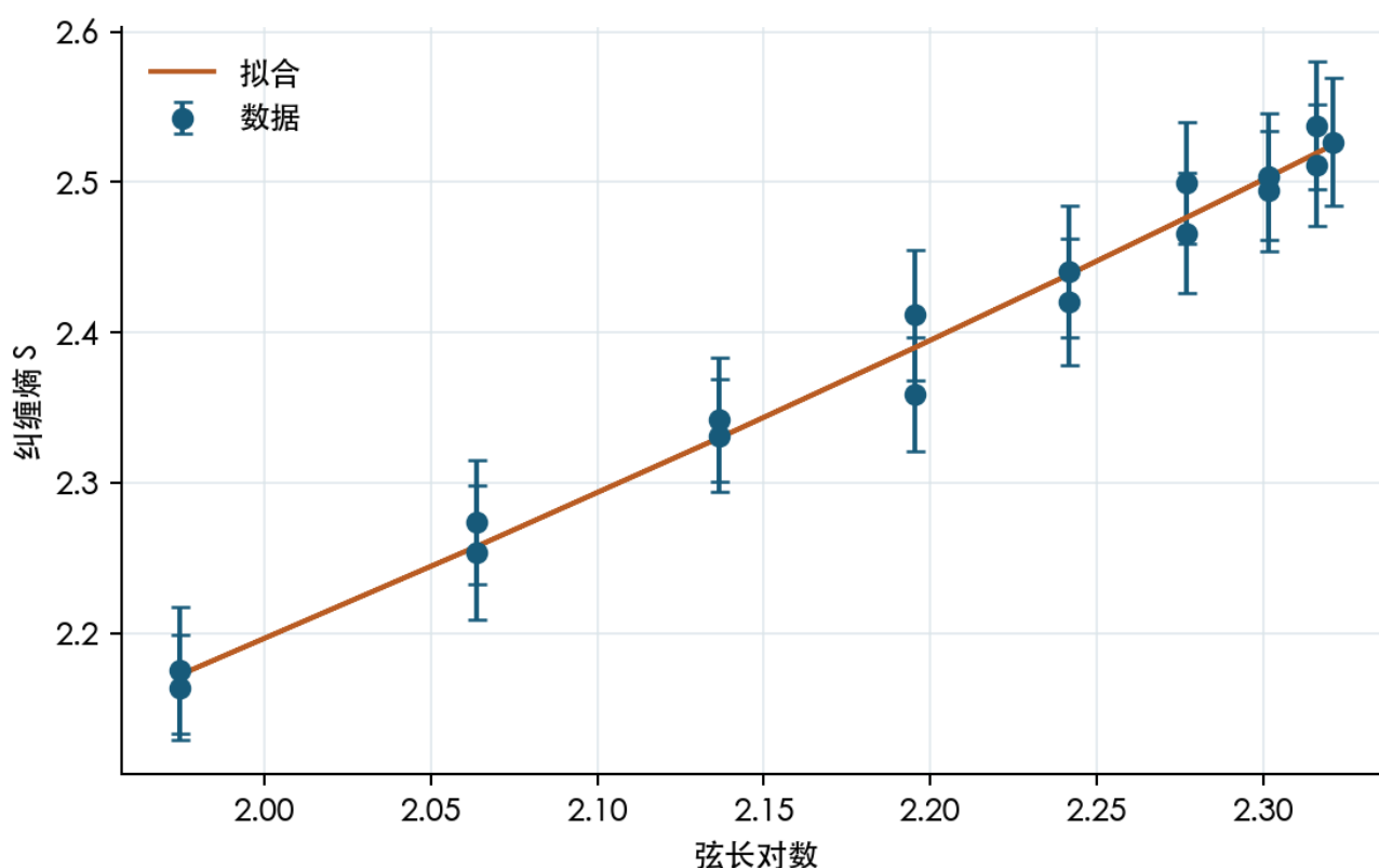
图 13. 选定 DIII 角度下纠缠熵对周期弦长的拟合。
