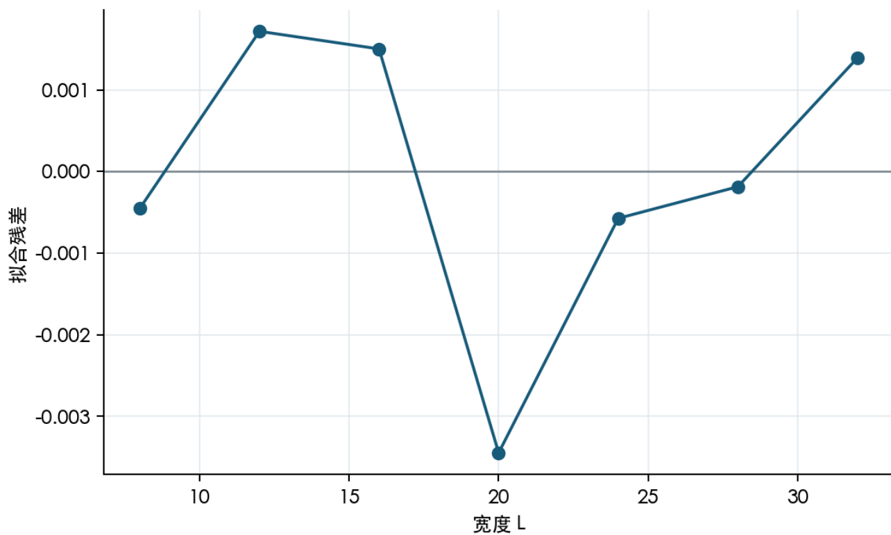
图 16. Casimir 有限尺寸拟合残差。 解读边界: 解读受有限宽度和预先声明拟合窗口约束。
