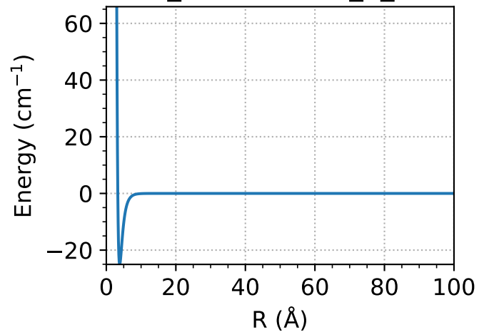
V_Lambda = 0_2_2
