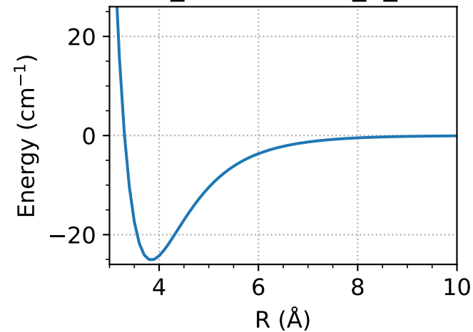
V_Lambda = 0_2_2
