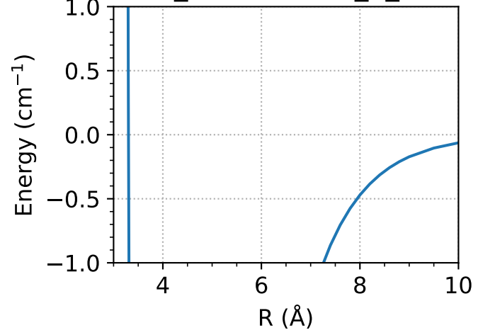
V_Lambda = 0_2_2
