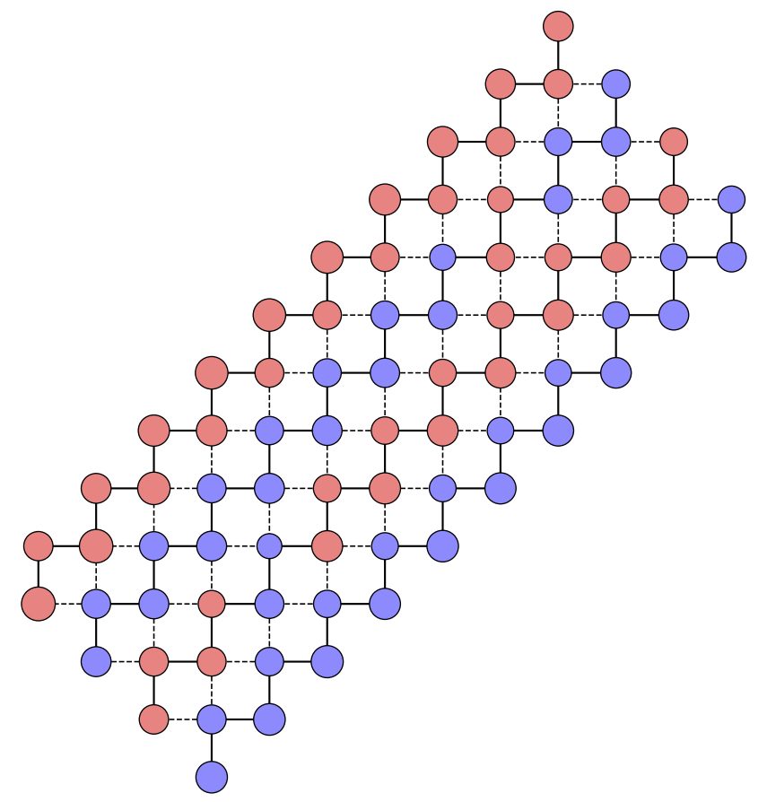
Layer 1 — itinerant electrons
