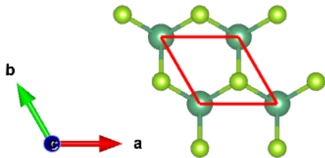
Original NbSe 2
