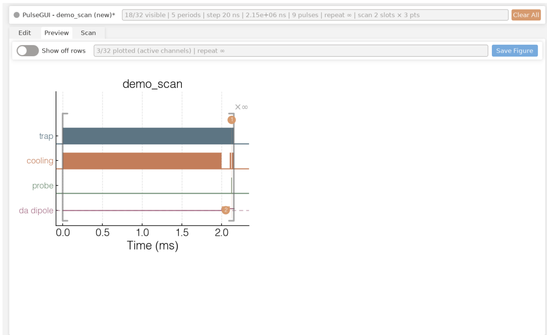
Figure 3.4: Preview 标签页的真实截图。画的是 未展开 的周期表；每条数字 channel 一行方波，模拟总线画成空心阶梯线。绑定 slot 的区间用贯穿所有行的半透明色带标出：duration 的标号在顶部、DAC 的在底部、delay 的在对应通道行，并带白色描边避免压字。
