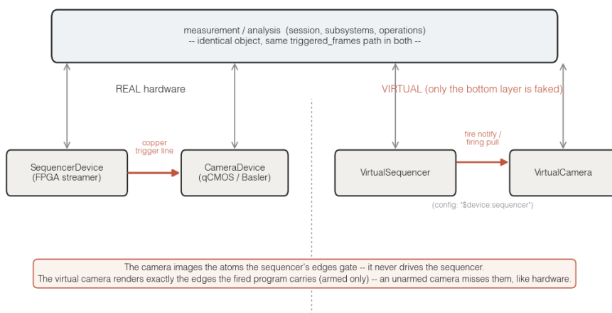
Figure 7.1: 虚拟 == 实机：只有最底层被仿真。 上方的 measurement / analysis 栈 (session / subsystems / operations, 含唯一编排 triggered\_frames ) 在真机与虚拟下是 同一个对象、走同一条代码路径 。真机里序列器用一根 铜触发线 接到相机；虚拟里 VirtualSequencer 的 fire 通知 / firing 拉取这根 被仿真的触发线 驱动 VirtualCamera (config 用 "\device:sequencer" 接线)。两边相机都 只按到达的触发边沿成像、从不驱动序列器 ；虚拟相机严格按 fired 程序在其触发线上 真实携带 的边沿数渲染帧， 未武装就漏掉边沿 ——和真机一模一样。所以换真机只改 connect() ，上面一行分析代码都不用动。
