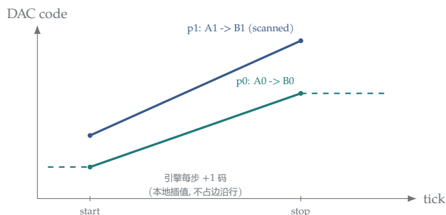
Figure 7.1: ramp 段: 引擎在 start/stop tick 之间本地线性插值。端点绑定 slot 时, 不同扫描点 (p0/p1) 画出不同起止——dual value_select 让一条段同时扫两个端点。
