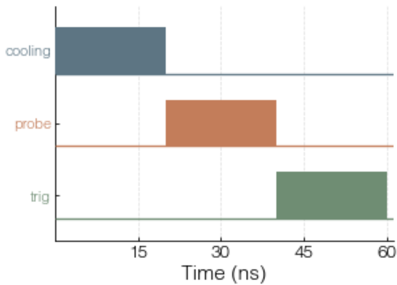
Figure 3.1: 前端脉冲实绘: 三路通道在相邻 20 ns tick 上背靠背切换——引擎的最小脉宽与分辨率就是 1 个 tick; 预取流水线让这些 1-tick 边沿逐拍打出, 中间无空拍。
