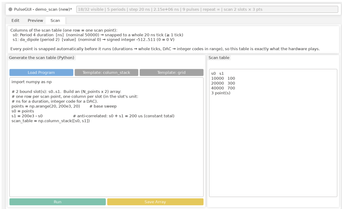
Figure 3.3: Scan 标签页的真实截图。顶部列出扫描表的各列（每个绑定的 slot 一列，含它绑的字段与单位）；代码框上方是 Load Program 与两个模板按钮，下方是 Run / Save Array 按钮；右侧是只读的扫描表预览。
