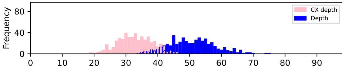
AG
