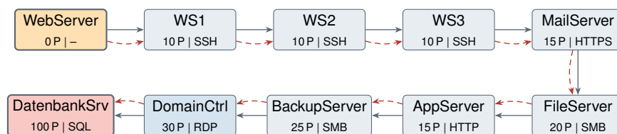
Abbildung 3.5: Topologie chain , verwendet für das Angreifertraining. Jeder Knoten gibt Erreichbarkeit und Zugangsdaten ausschließlich für seinen Nachfolger preis; von dieser Topologie führen neun Sprünge bis zum Crown Jewel.
