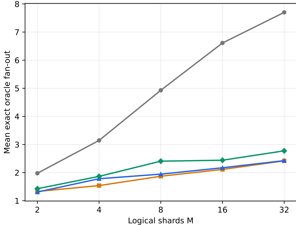
GloVe-200
