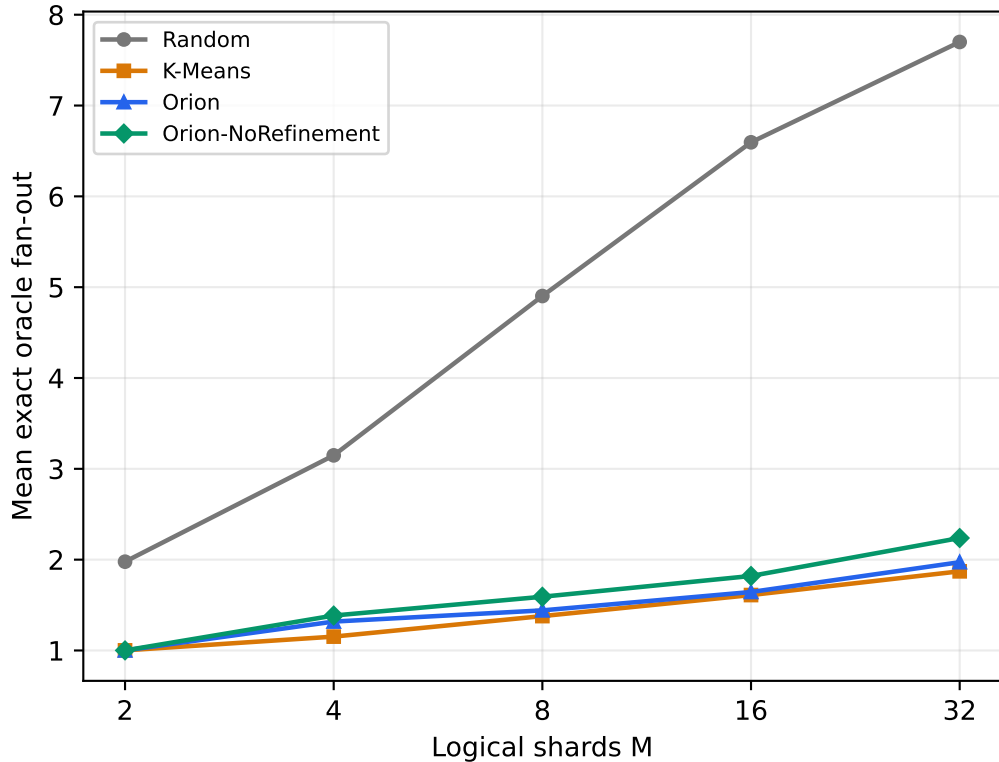
SIFT1M
