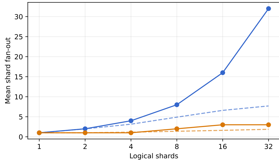
SIFT1M
