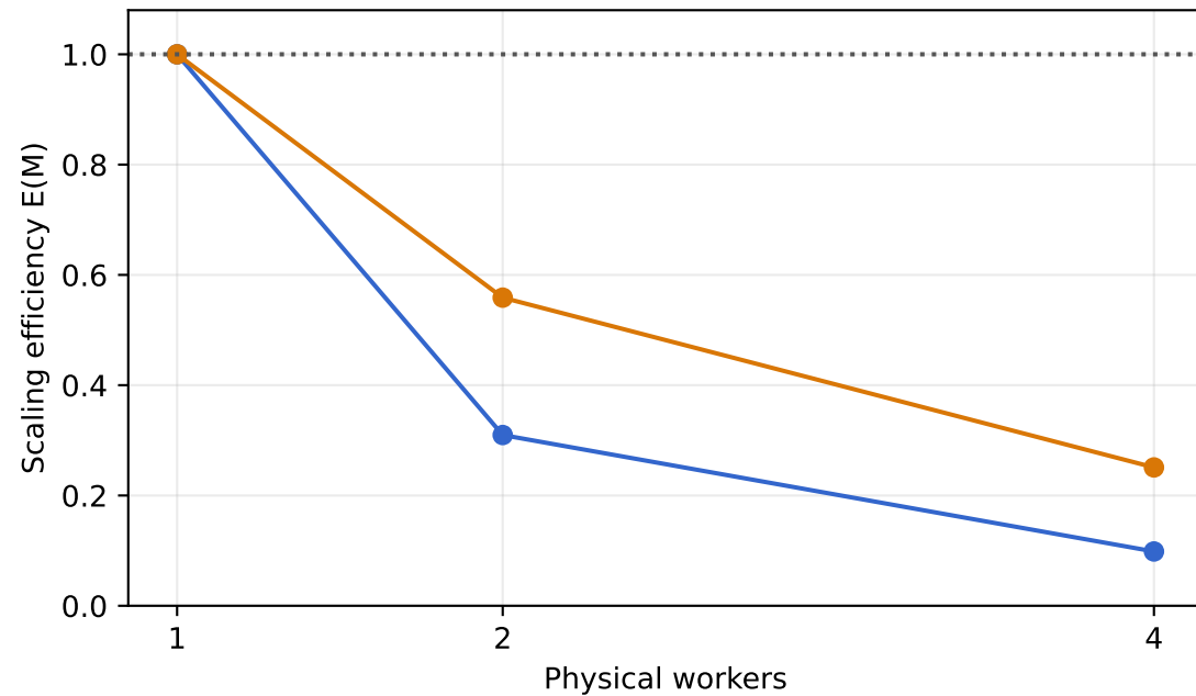
SIFT1M
