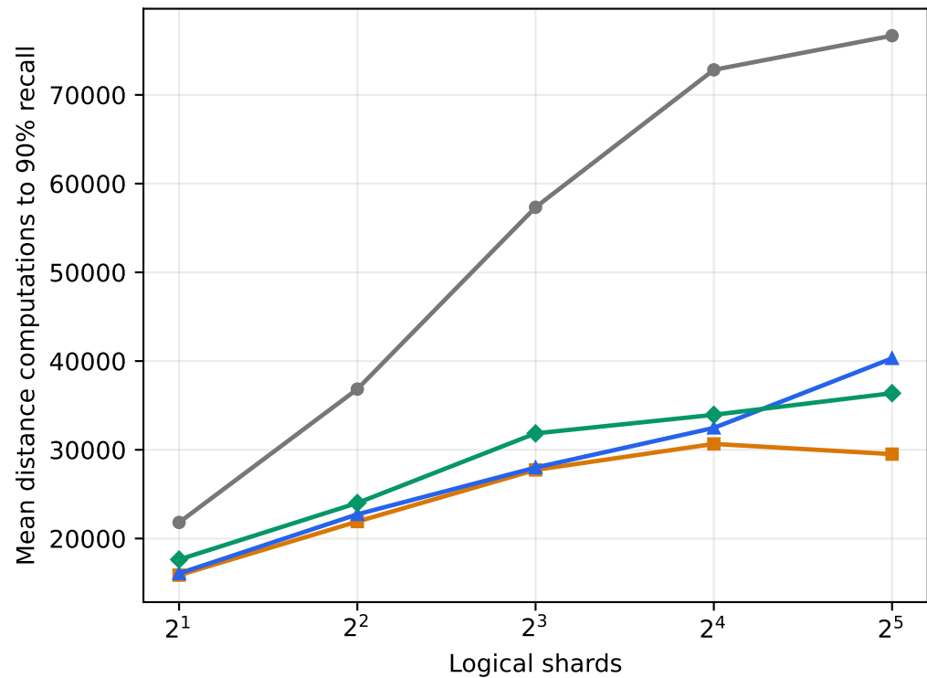
GloVe-200
