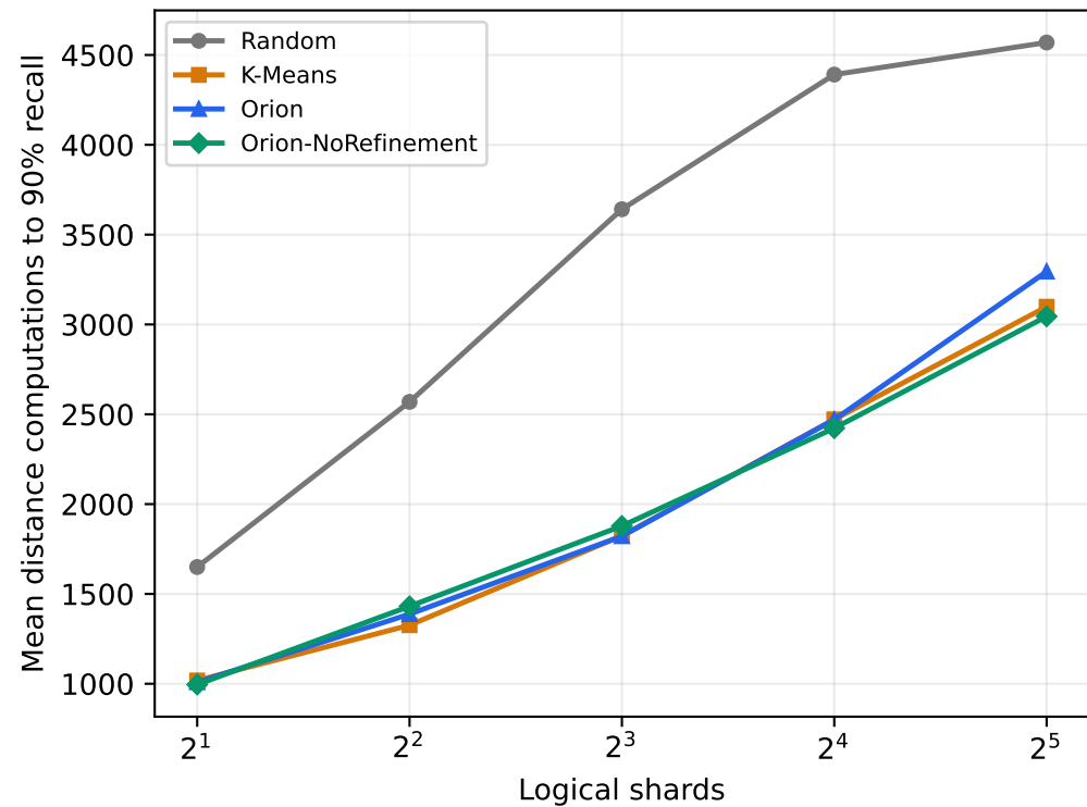
SIFT1M
