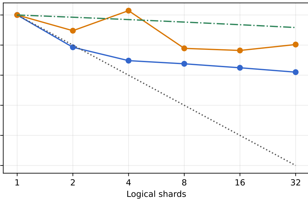
SIFT1M
