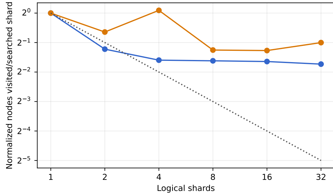
SIFT1M
